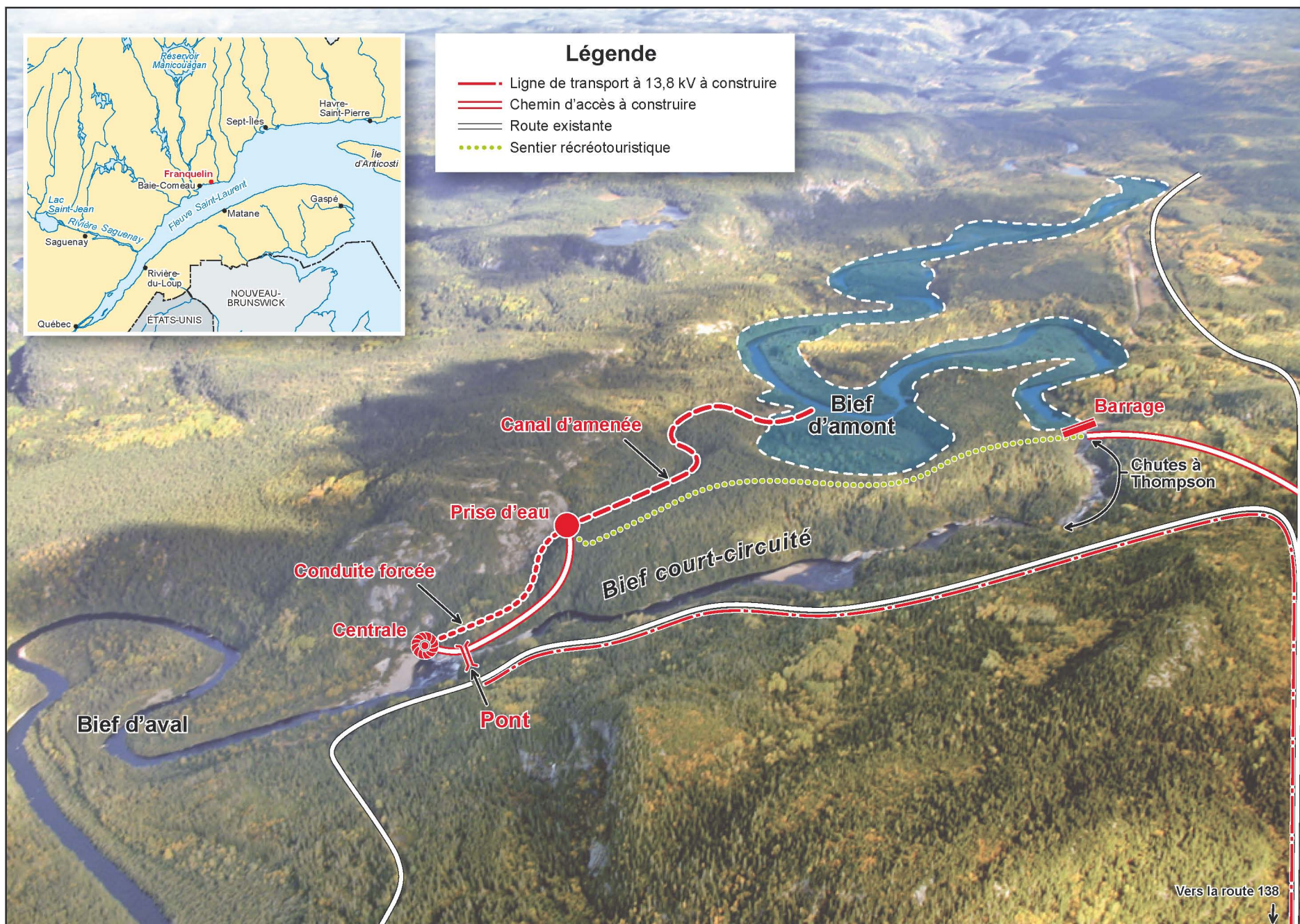
Figure 1 Aménagement hydroélectrique des chutes à Thompson sur la rivière Franquelin
