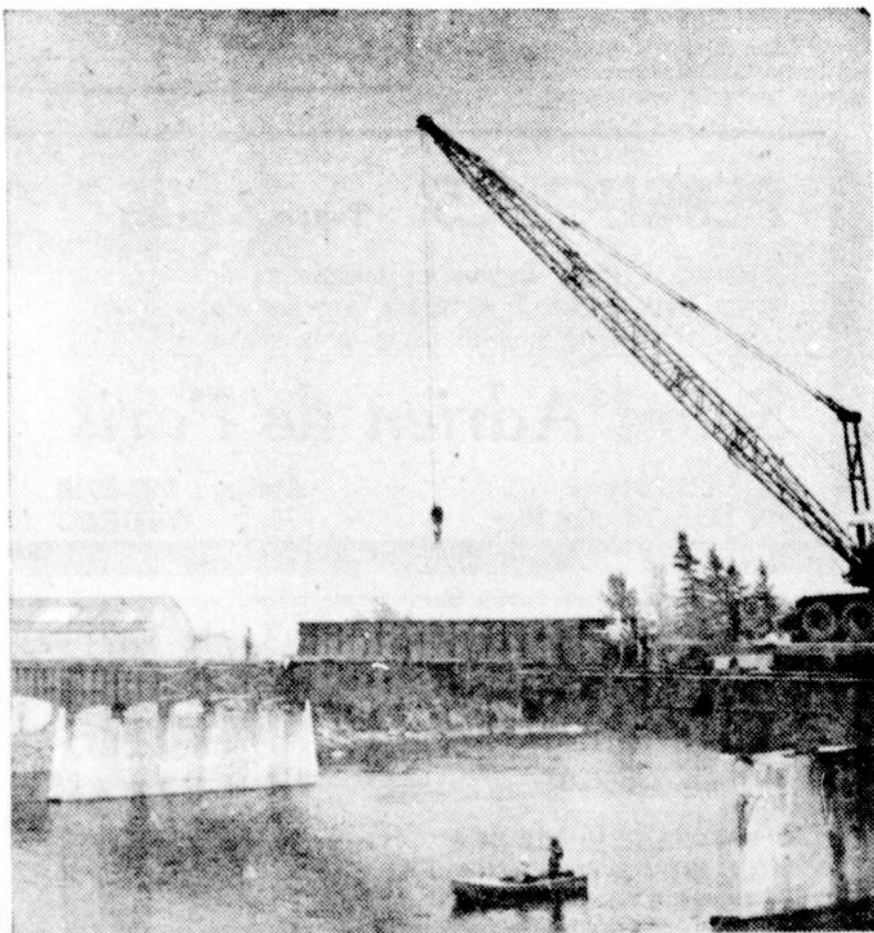
CA S'EST PASSE AU PONT DE LA RIVIERE DU-SUD - C'est de la Poutre aux yeux... Une poutre d'acier de 7 tonnes, une grue de 40 tonnes et Arco Construction qui travaille sur un projet de 530 mille dollars. Ça fait une bonne photo, pas vrai?
