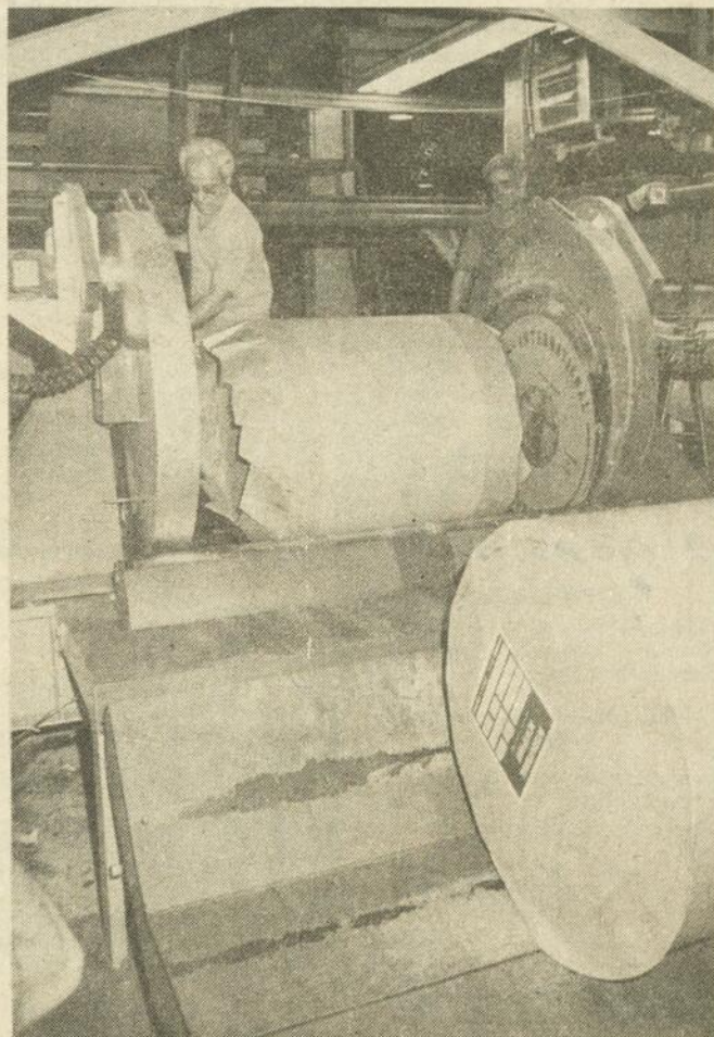
Grâce aux améliorations apportées à la ligne d'emballage automatique de l'usine de la CIP à Trois-Rivières, toute la production de papier-journal sera désormais emballée automatiquement. Un système computer, jumelé à la ligne existante, est chargé de coordonner toutes les opérations d'emballage. (Photo Michel Brière)
