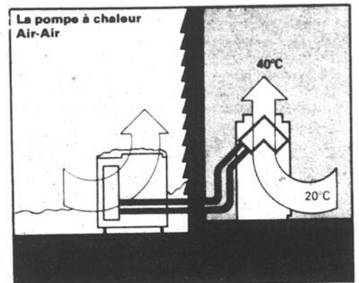
La pompe à chaleur eau-air extrait la chaleur de l'eau puisée dans le sous-sol avant de la rejeter dans un bassin d'infiltration.
