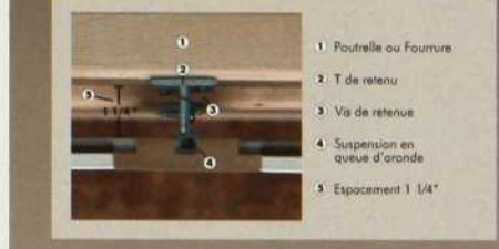
Coupe de suspension
