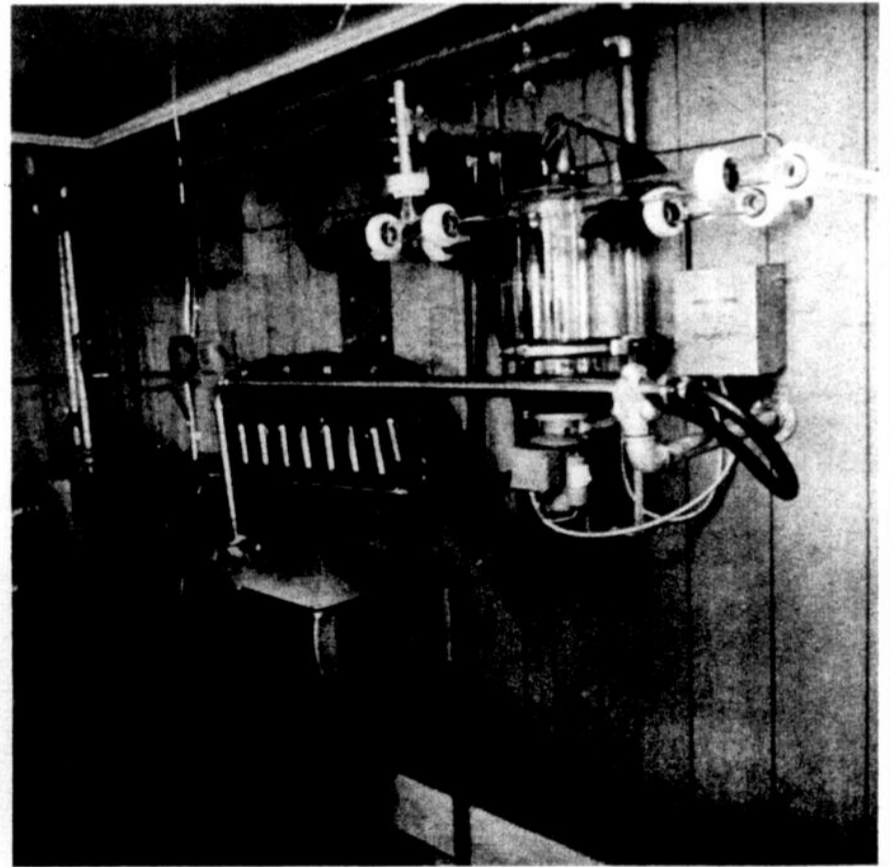
Le centre nerveux de système Comatic est le groupe récepteur, compact, économique, efficace et, par-dessus tout, de prix concurrentiel. On monte la pompe centrifuge directement sous la jarre de réception du lait. La trappe et les supports de filtre font aussi partie de l'unité.
