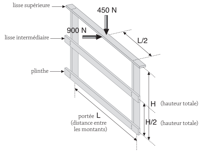
Charges concentrées
