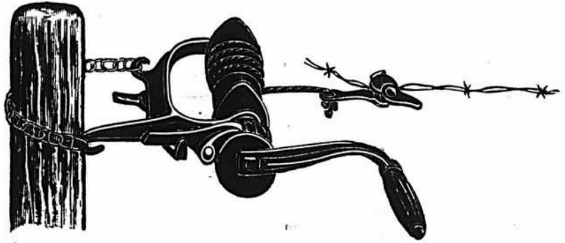
Extracteur de crampes et outil à épissures.
