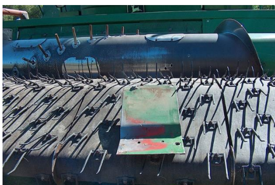
Figure 11-6. Plaque déflectrice du convoyeur.
