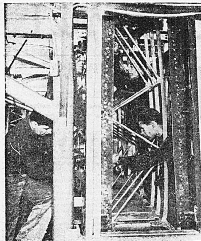
Des ouvriers de l'usine Boeing Aircraft, à Seattle, Washington, procèdent à la construction de l'une des forteresses volantes de 2 tonnes qui seront livrées sous peu à la Grande-Bretagne. Ces bombardiers peuvent transporter cinq tonnes et demie d'explosifs et filer à une vitesse de 280 milles à l'heure.
