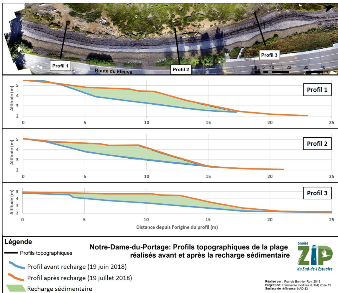
Figure 10. Profils topographiques de la plage réalisés avant après la recharge sédimentaire
