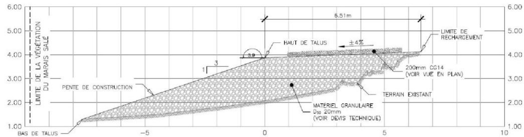
PROFIL EN TRAVERS - 0+060
