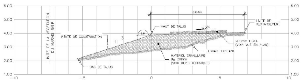
PROFIL EN TRAVERS - 0+180
