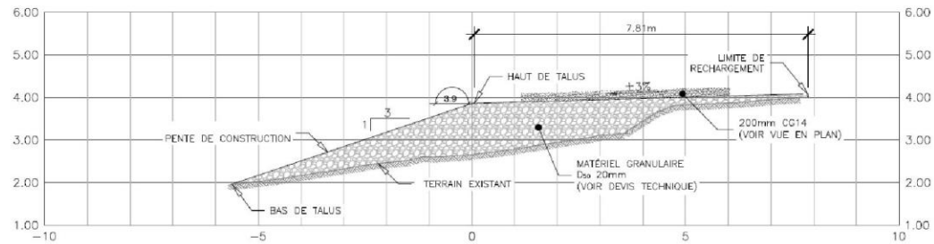
PROFIL EN TRAVERS - 0+140
