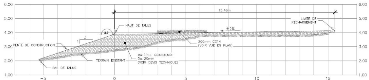
PROFIL EN TRAVERS - 0+160
