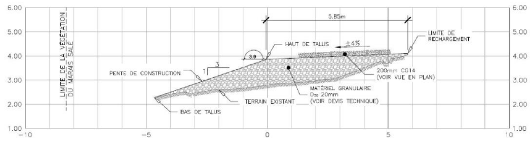
PROFIL EN TRAVERS - 0+170
