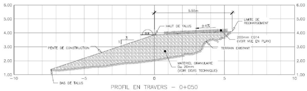
PROFIL EN TRAVERS - 0+050
