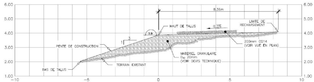
PROFIL EN TRAVERS - 0+120
