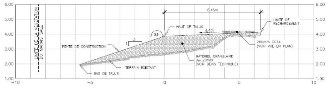
PROFIL EN TRAVERS - 0+150
