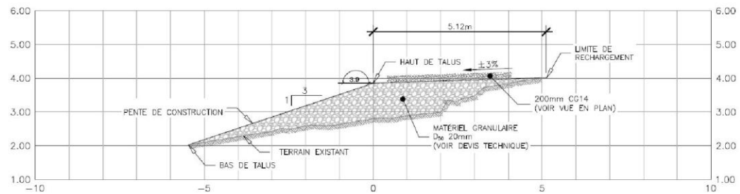
PROFIL EN TRAVERS - 0+130
