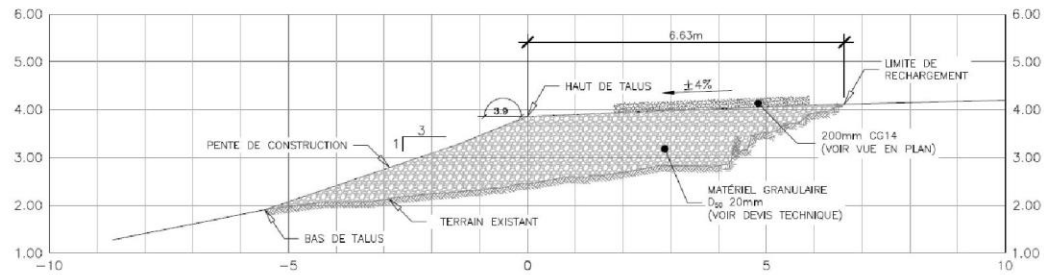
PROFIL EN TRAVERS - 0+010
