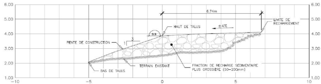
PROFIL EN TRAVERS - 0+001
