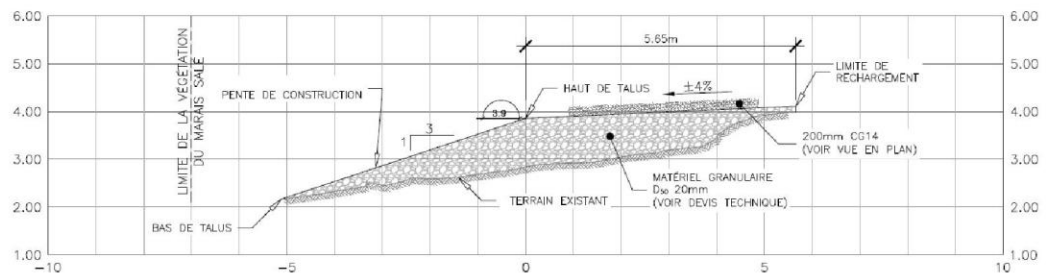
PROFIL EN TRAVERS - 0+189
