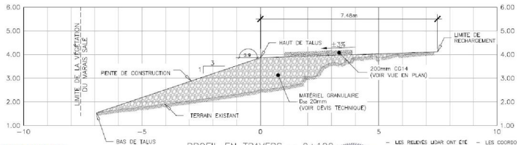
PROFIL EN TRAVERS - 0+100
