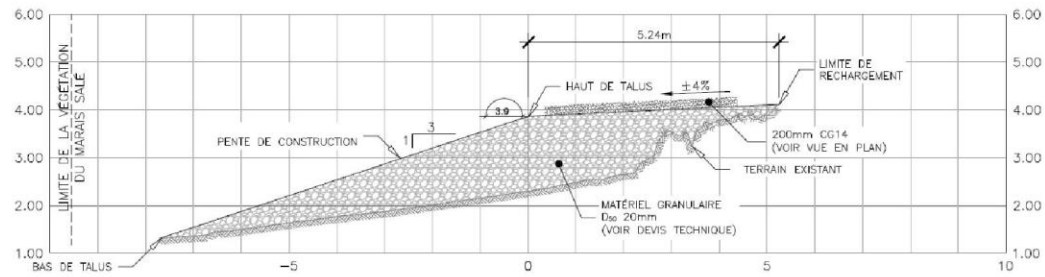
PROFIL EN TRAVERS - 0+070
