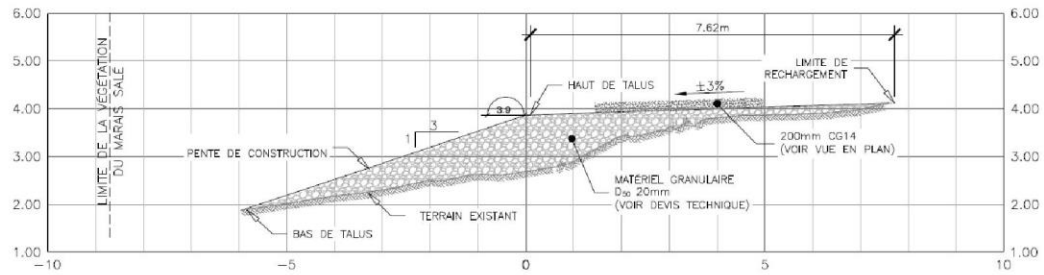
PROFIL EN TRAVERS - 0+110
