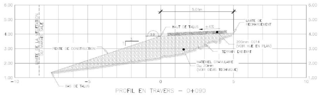
PROFIL EN TRAVERS - 0+090
