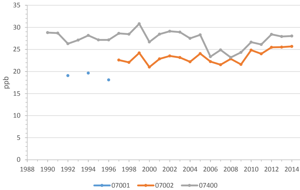
Figure 5 Concentrations annuelles d'ozone
