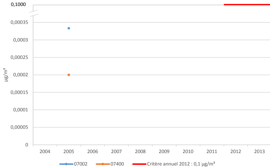
Figure 18 Concentrations annuelles de cobalt dans les particules en suspension
