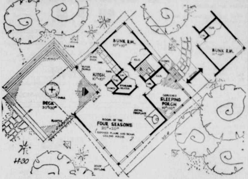
Plan du H-30 : La maison est de 718 pieds carrés et la véranda de 100 pieds carrés. Les dimensions, sans la galerie, sont de 30'4" par 30'4".
