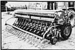
Semoir Hassia 26 disques doubles, marqueurs, herse arrière
