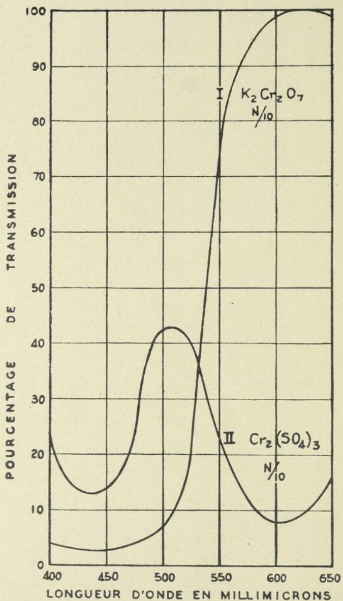
FIG I.-SPECTRES D'ABSORPTION DE SOLUTIONS DECINORMALES DE BICHROMATE DE POTASSIUM (I) ET DE SULFATE DE CHROME TRIVALENT (II)
