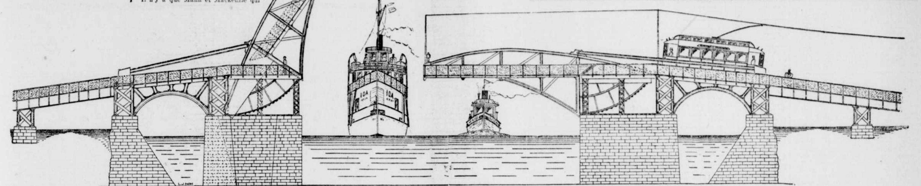
Projet soumis au gouvernement fédéral, par M. François Lapointe, d'un pont sur le canal Lachine, à St Henri. Ce pont aura deux voies pour chars électriques, deux pour voitures et deux pour piétons. Ce système de construction est tout ce qu'il y a de plus moderne.
