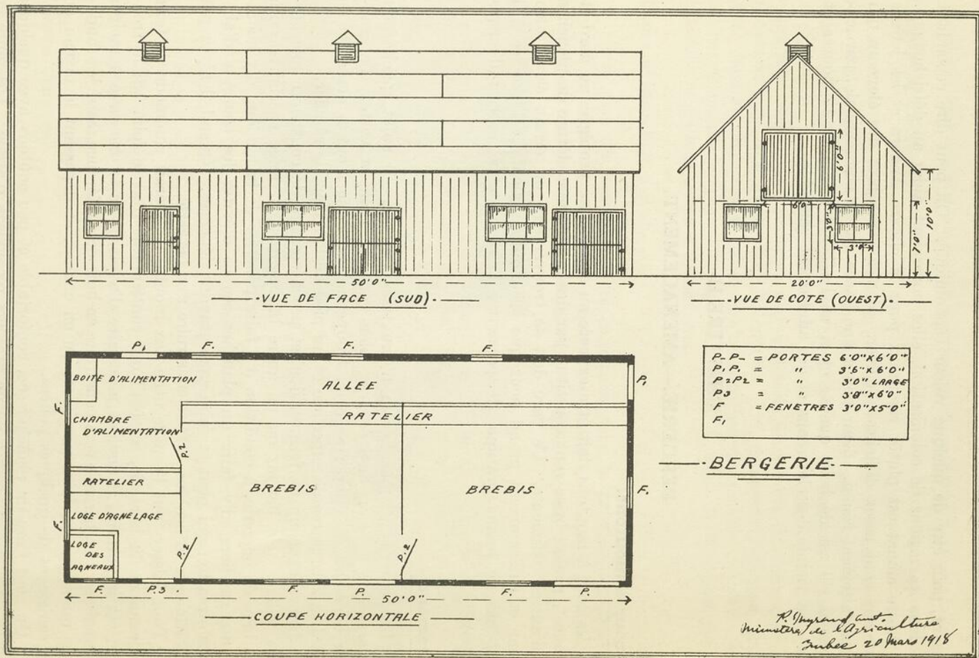
Plan d'une bergerie pour un troupeau ordinaire sur une ferme.
