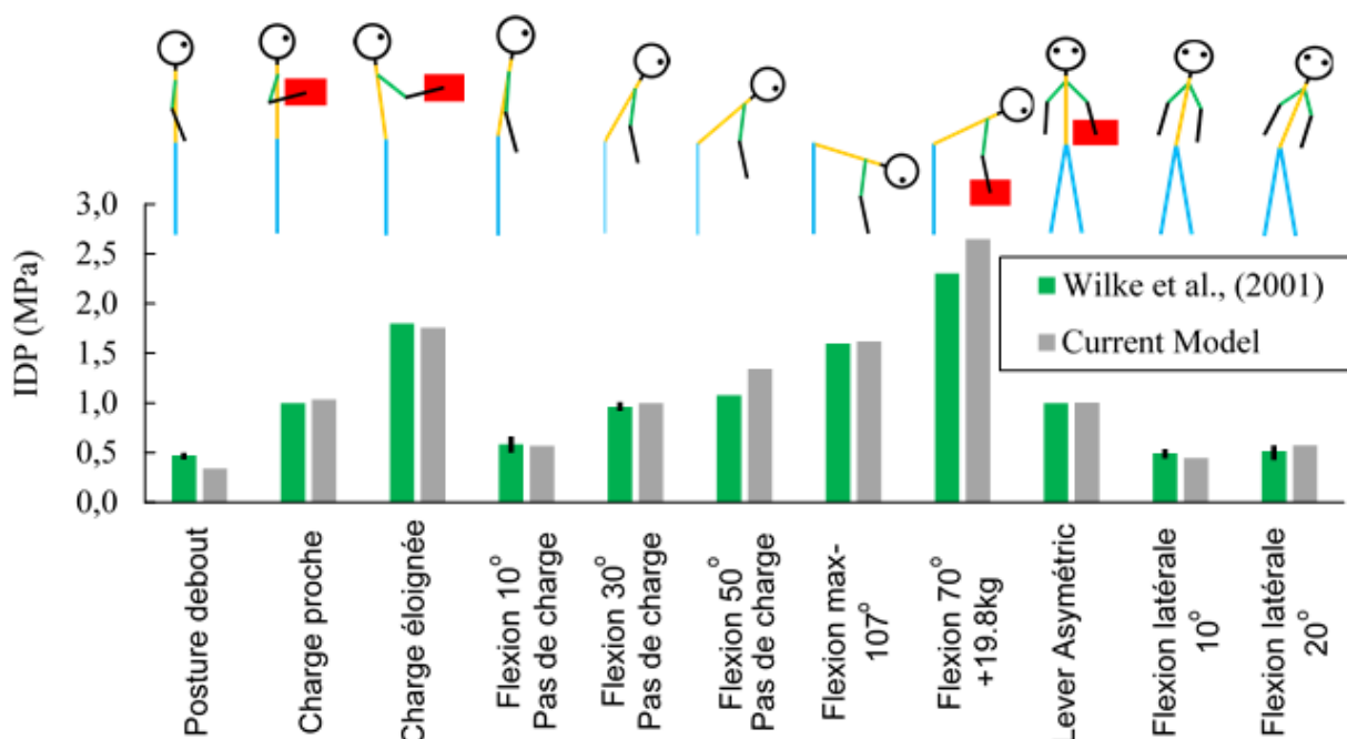
Figure 4-3. Pressions intradiscales mesurées par rapport à ceux calculées du modèle au niveau L4-L5; le modèle est personnalisé ici pour correspondre aux paramètres personnels du sujet ayant participé à l'étude in vivo de Wilke et al (2001) : sexe = homme, âge = 45 ans, Poids = 72 kg et Taille = 173,9 cm.
