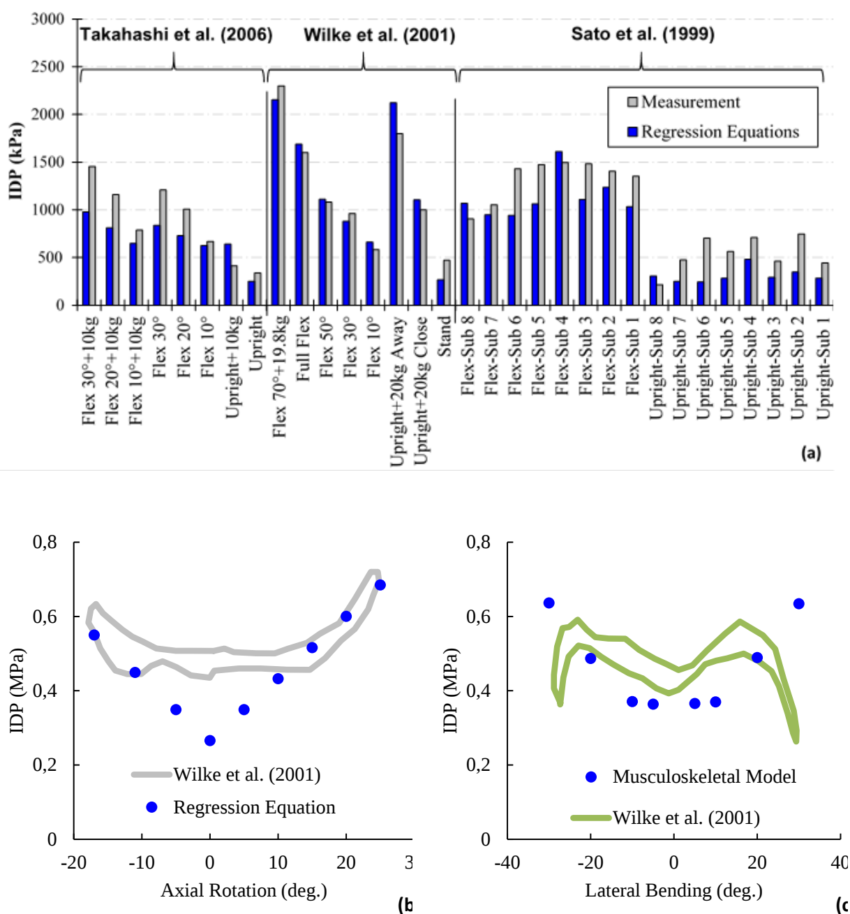
Figure 7-2. Pressions intradiscales (IDP) estimées à partir des équations de régression (a et b) et du modèle MS (c), par rapport aux mesures lors de tâches sagittales symétriques (a; Flex = flexion : Sub = Sujet; Sato et al. , (1999) ont mesuré le IDP de 8 sujets), la rotation axiale (b) et la flexion latérale (c; les équations de régression proposées ne permettent pas d'estimer les charges vertébrales en flexion latérale pure; nous avons donc utilisé le modèle MS pour estimer ces charges.)
