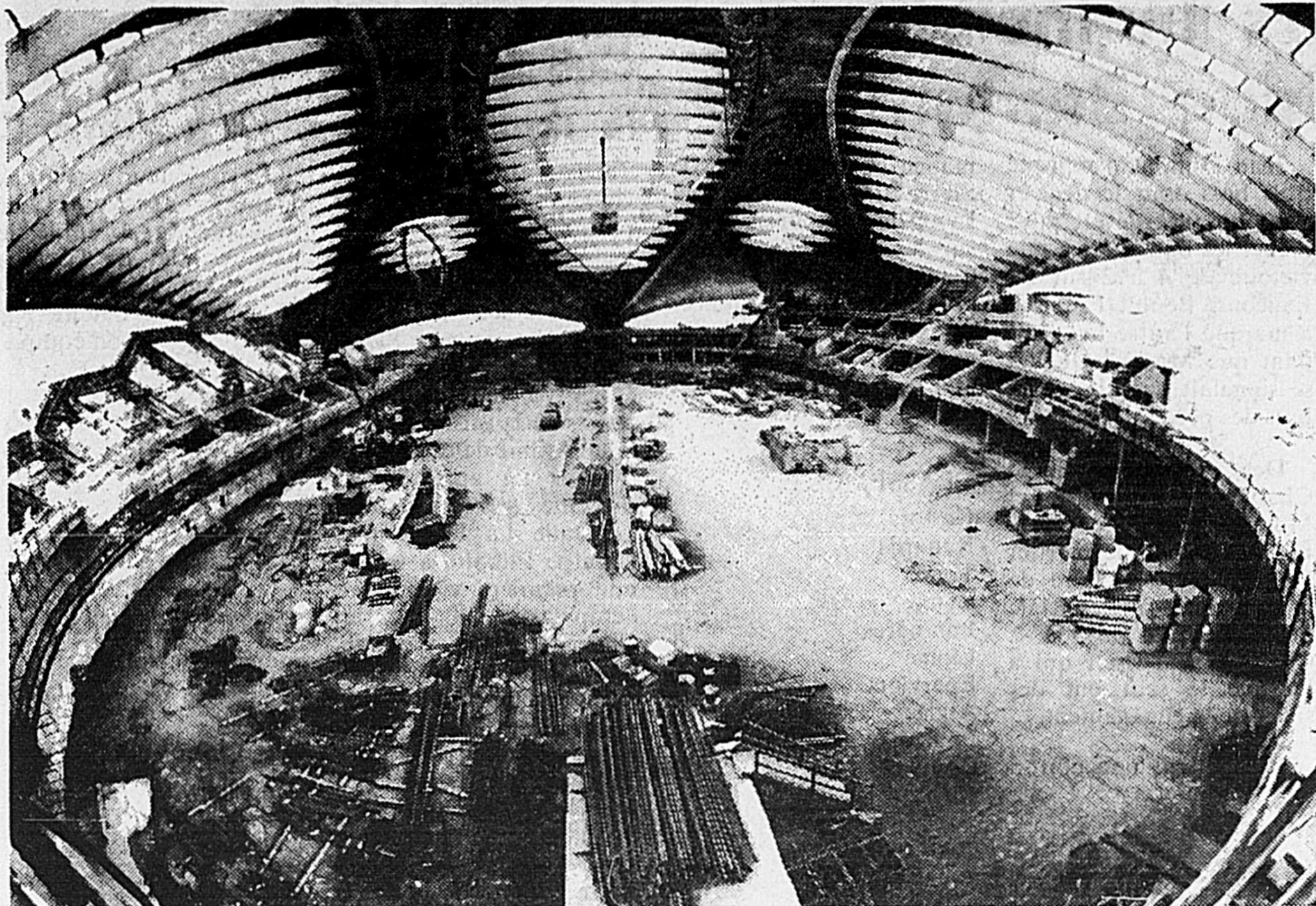
Les ouvriers commencent à monter la piste et les gradins du Vélodrome où auront lieu les épreuves olympiques de cyclisme et de judo.
