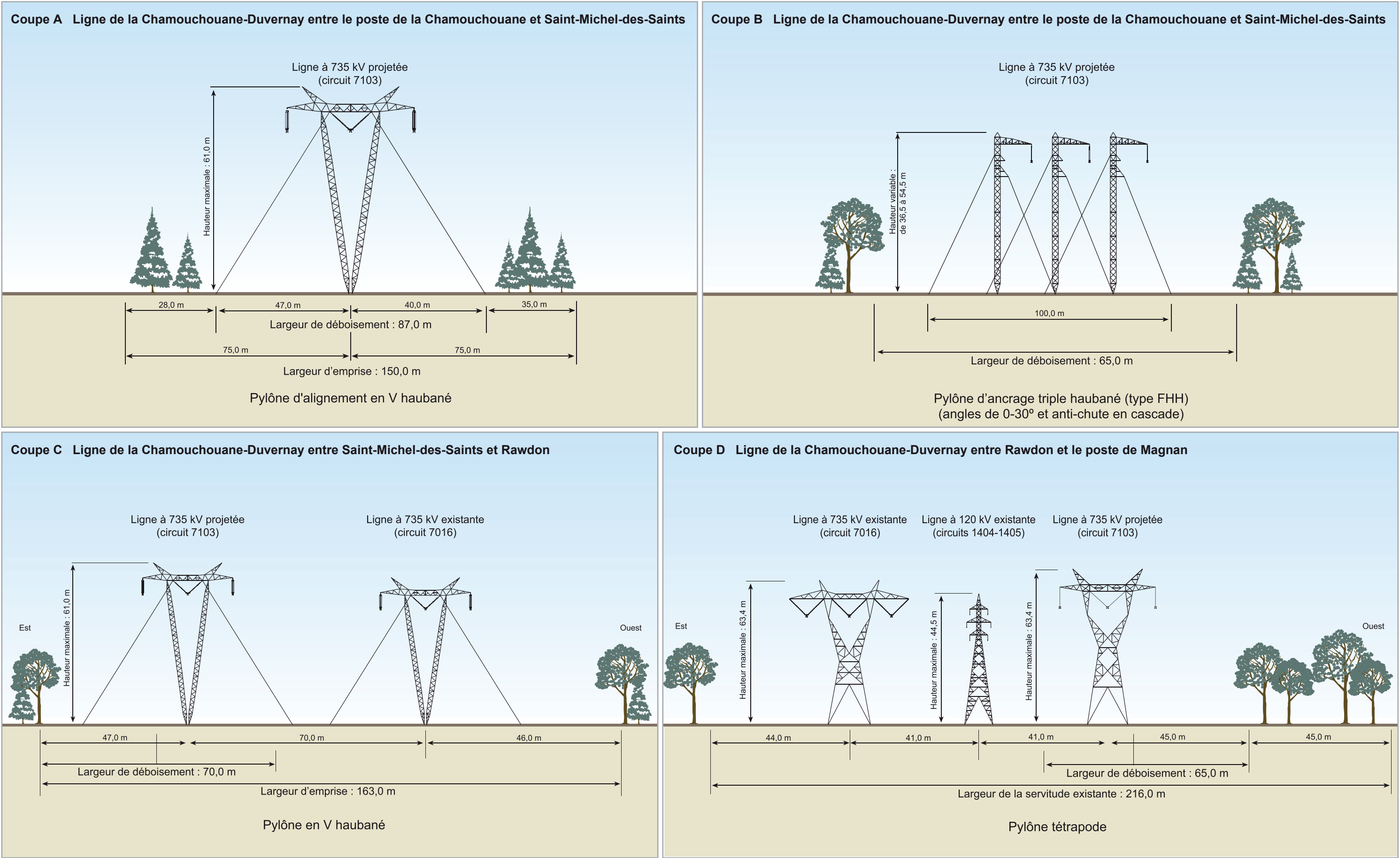
Figure 5 Les supports et les emprises types de la ligne et de la déviation projetées – Coupes A à D
