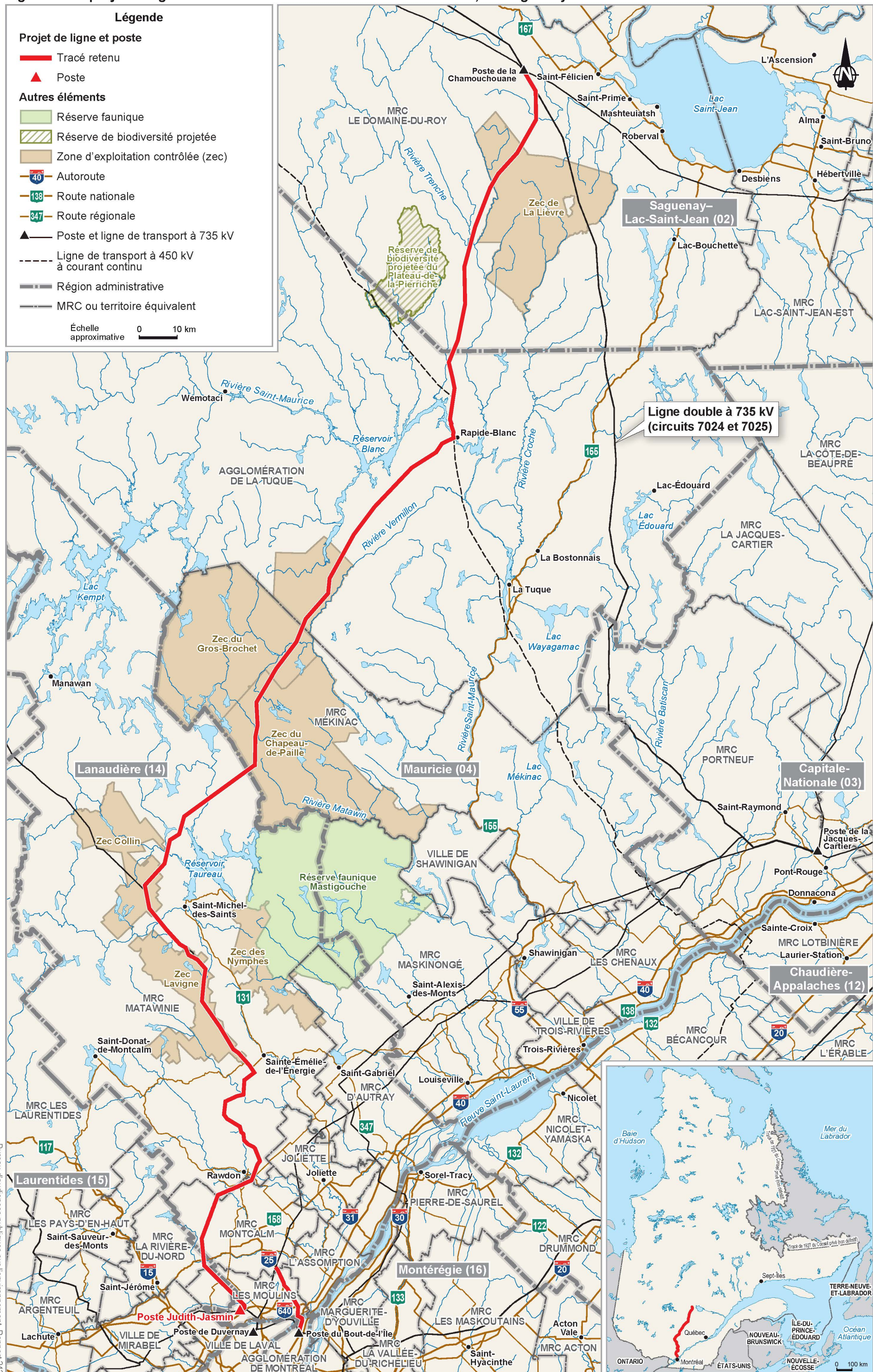
Figure 1 Le projet de ligne à 735 kV de la Chamouchouane–Bout-de-l'Île, du Saguenay–Lac-Saint-Jean à Montréal
