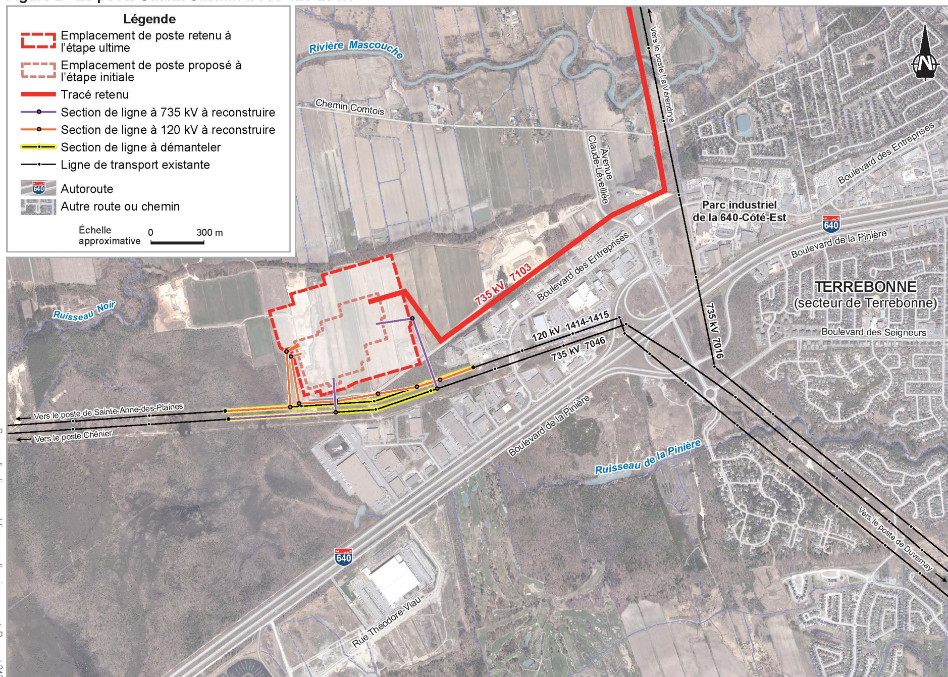
Figure 2 Le poste Judith-Jasmin à 735-120-25 kV
