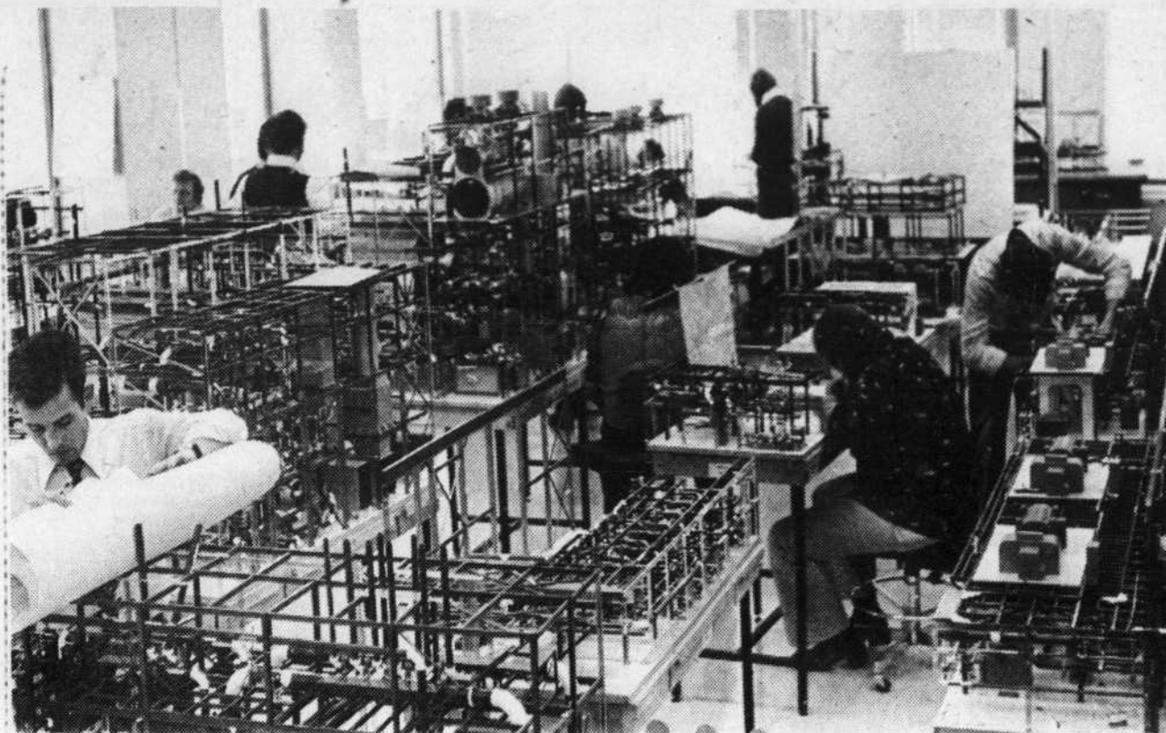
Quelque 40.000 heures-homme ont été requises à la fabrication du modèle qui apparaît ci-haut d'une centrale qui alimentera en énergie électrique et en vapeur le projet Synchrone. Monenco réalise la totalité de l'ingénierie et de l'approvisionnement pour cette centrale qui sera une des plus importantes du genre dans le monde.
