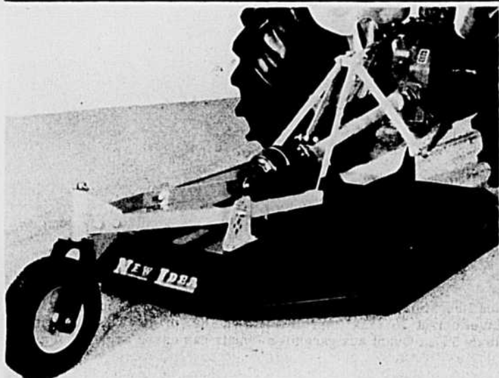
La compagnie New Idea vient de mettre sur le marché cette nouvelle faucheuse rotative, la 452. La largeur de coupe est de 60 pouces tandis que sa hauteur minimum de coupe est de 1 1/2 pouce
