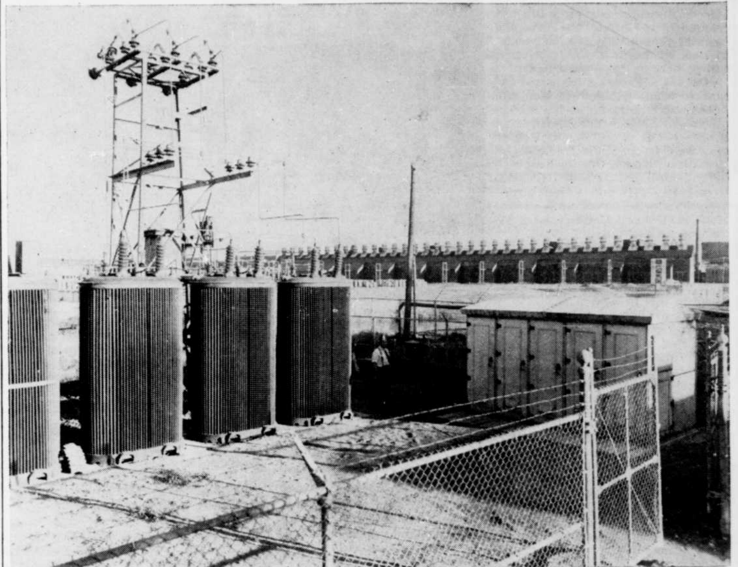
La sous-station de la Compagnie Électrique du Saguenay située rue Volta près de la route Taschereau. A gauche, on voit les transformateurs et à droite le kiosque des interrupteurs automatiques. Au centre, M. Armand Ouellet, employé de la Compagnie, en charge du service et de la patrouille des lignes dans les limites d'Arvida.
