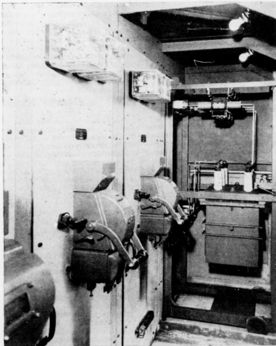
Vue intérieure du kiosque montrant un disjoncteur à l'huile, ouvert. A remarquer les relais de surcharge placés au-dessus des contrôles manuels.
