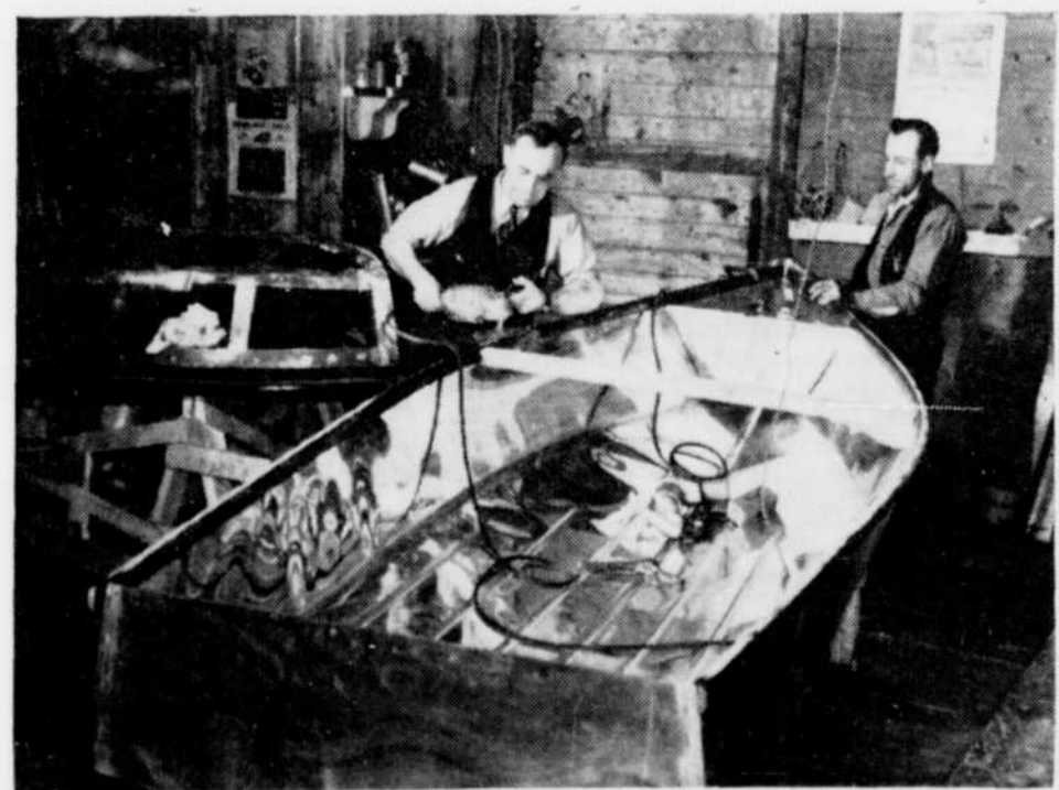
MM. Albert Trottier, contremaître et Laurent Gauthier, mettant la dernière main à l'une des fameuses chaloupes en aluminium construites par Les Produits d'Aluminium de Chicoutimi.
