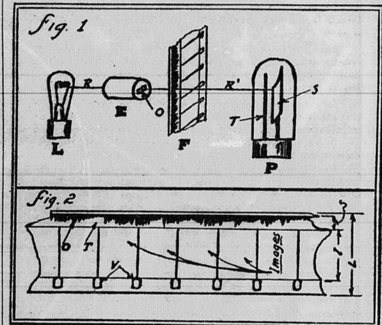
FIG. 1 — L—Lampe excitatrice de la cellule photo-électrique. S—Marge pour l'enregistrement du son. V—Trous pour permettre de dérouler le film. T—Espace transparent. O—Espace opaque.
