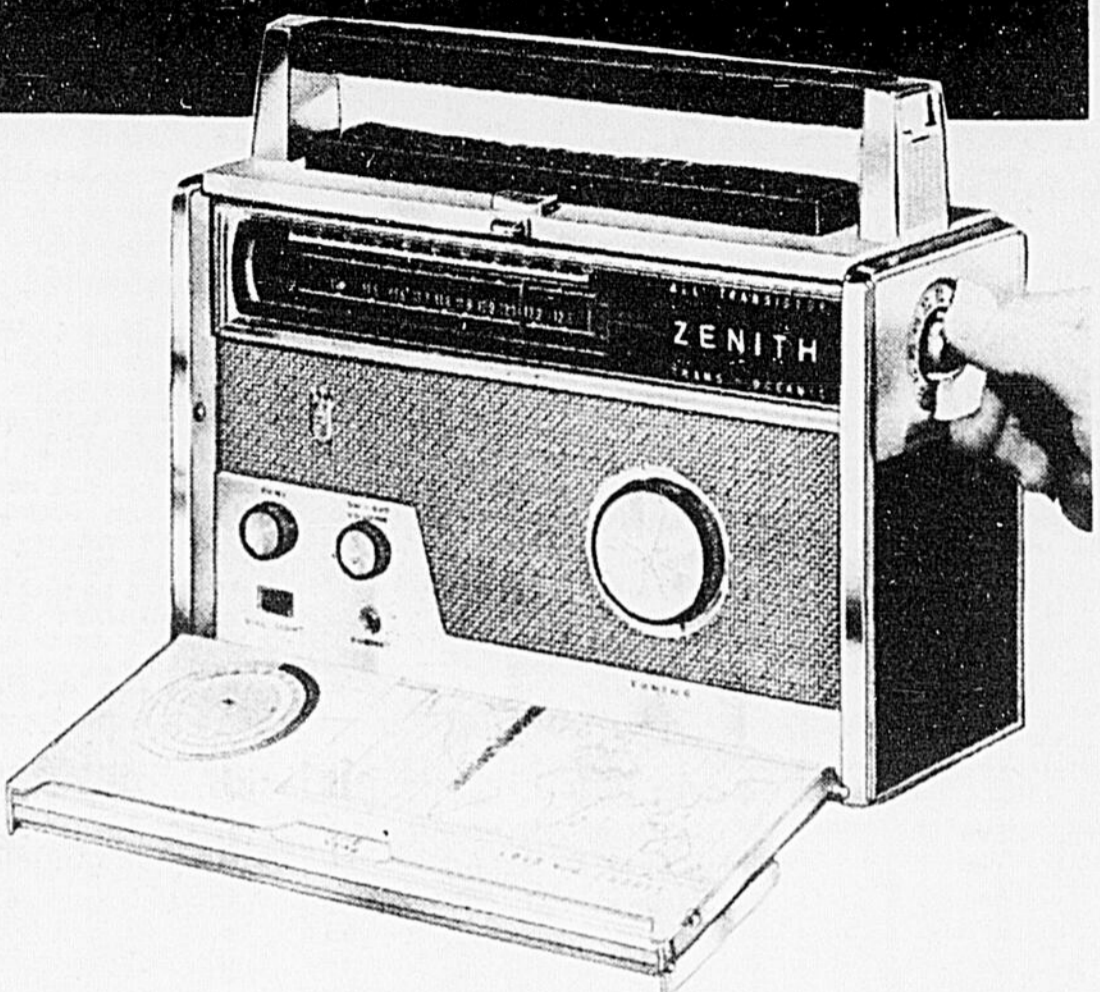
TRANS-OCEANIC TOUT TRANSISTOR Syntonisateur de station rotatif Contrôles de volume et tonalité indépendants Haut-parleur de haute qualité Antenne pour onde courte
