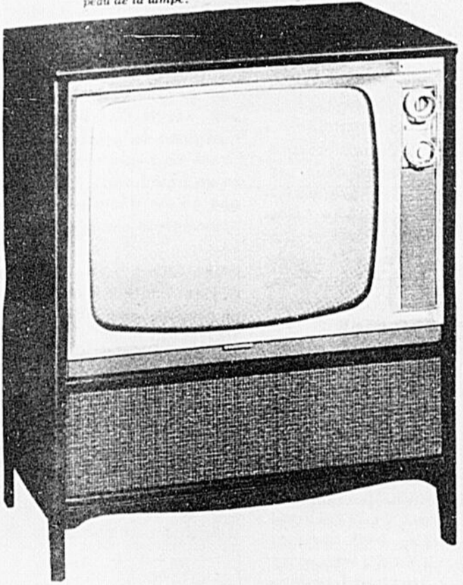
Le ROXBURY - Modèle M2735 Magnifique console de style transitionnel, fini noyer. Nouveau syntonisateur "Custom Video Range". Cadran VHF "Spotlite". Puissance d'image de 21,000 volts. Dimensions: hauteur 33", largeur 27 1/4", profondeur 17 1/4".
