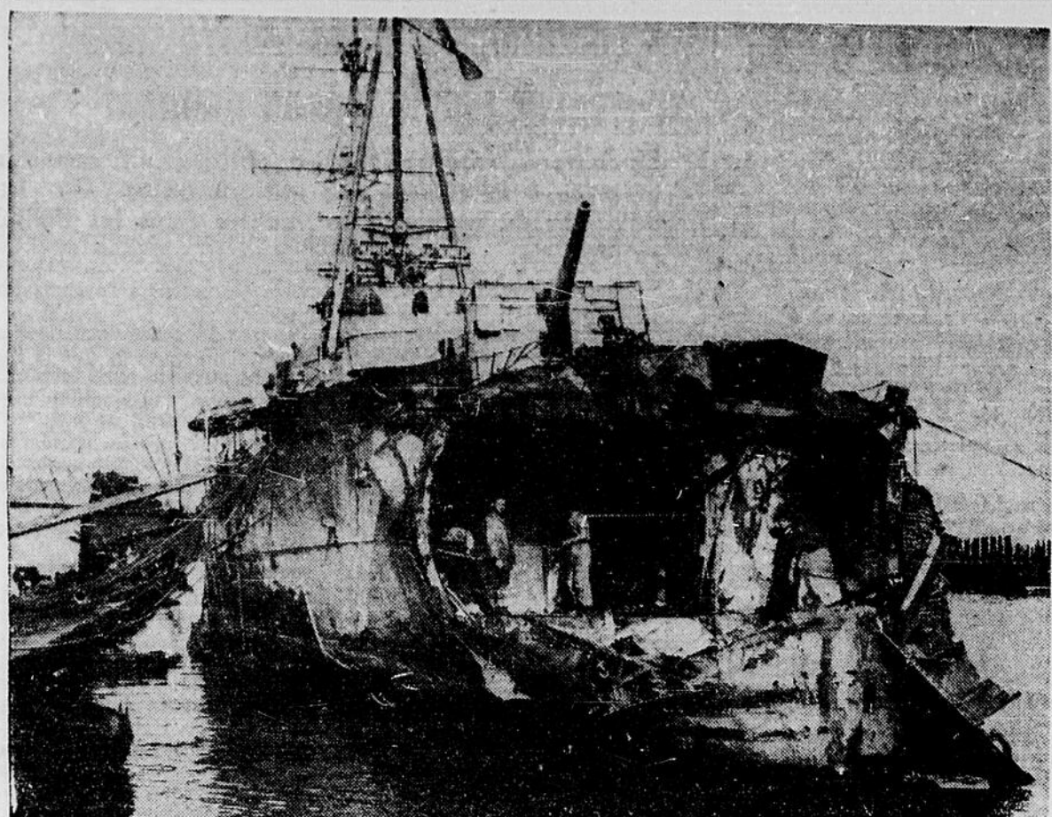
Ce trou béant à la poupe du croiseur britannique H.M.S. DELHI est l'oeuvre d'une bombe allemande, lancée au cours d'opérations navales au large de la côte nord-africaine en 1942. Bien que cette photo ne fut pas publiée avant aujourd'hui, le DELHI a repris la mer il y a deux ans.
