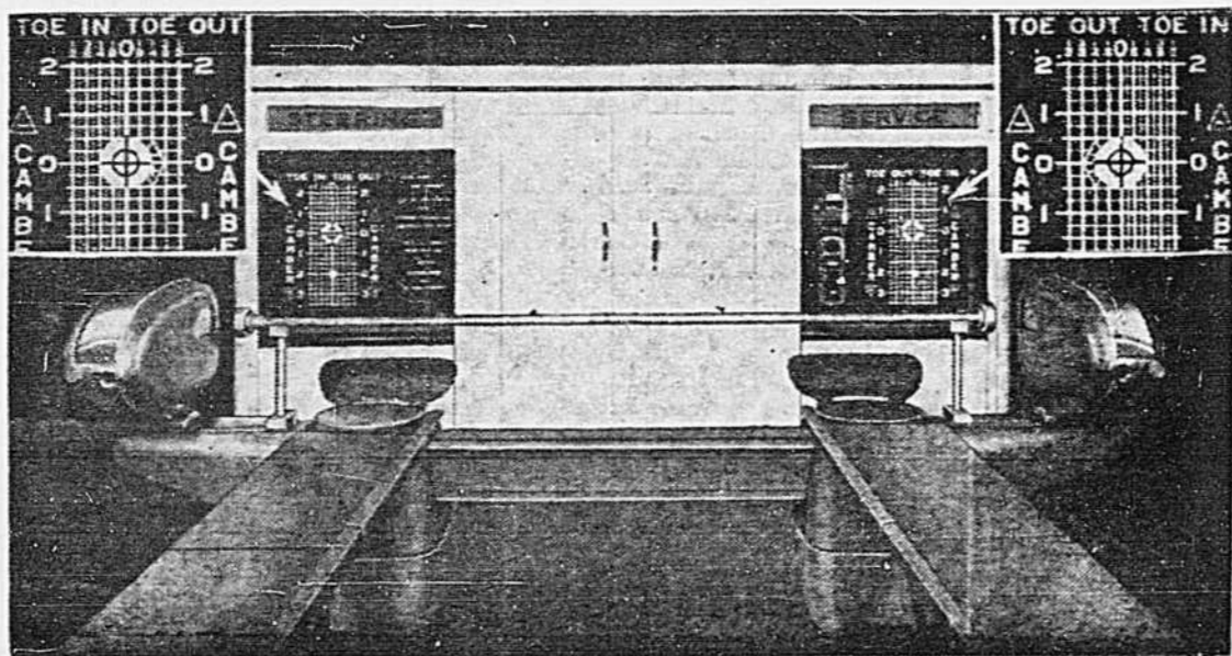
"VISUALINER" la méthode parfaite pour l'alignement et la correction des roues de votre véhicule
