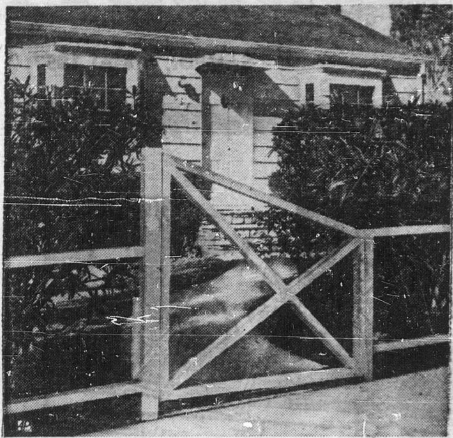
La simplicité distingue cette élégante clôture qui délimite la propriété. Facile à construire, elle est formée de 2 par 4 qui s'étendent entre ces poteaux de 4 par 4.
