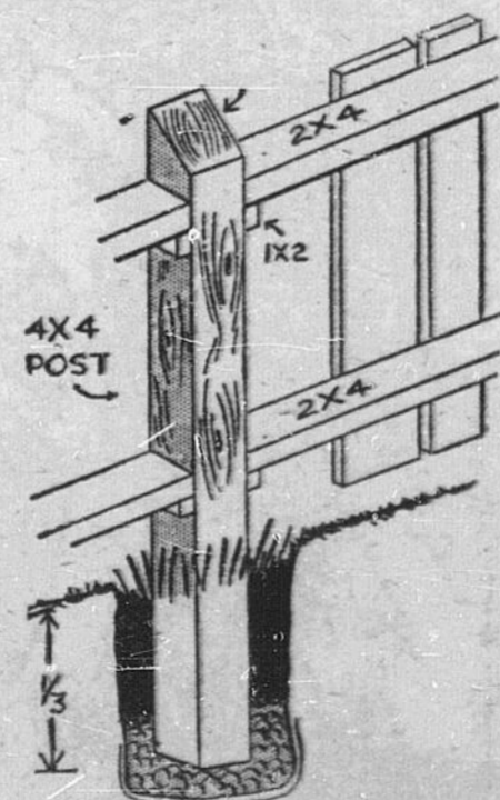
Plantez un tiers du poteau dans la terre. Coupez la tête en biseau.
