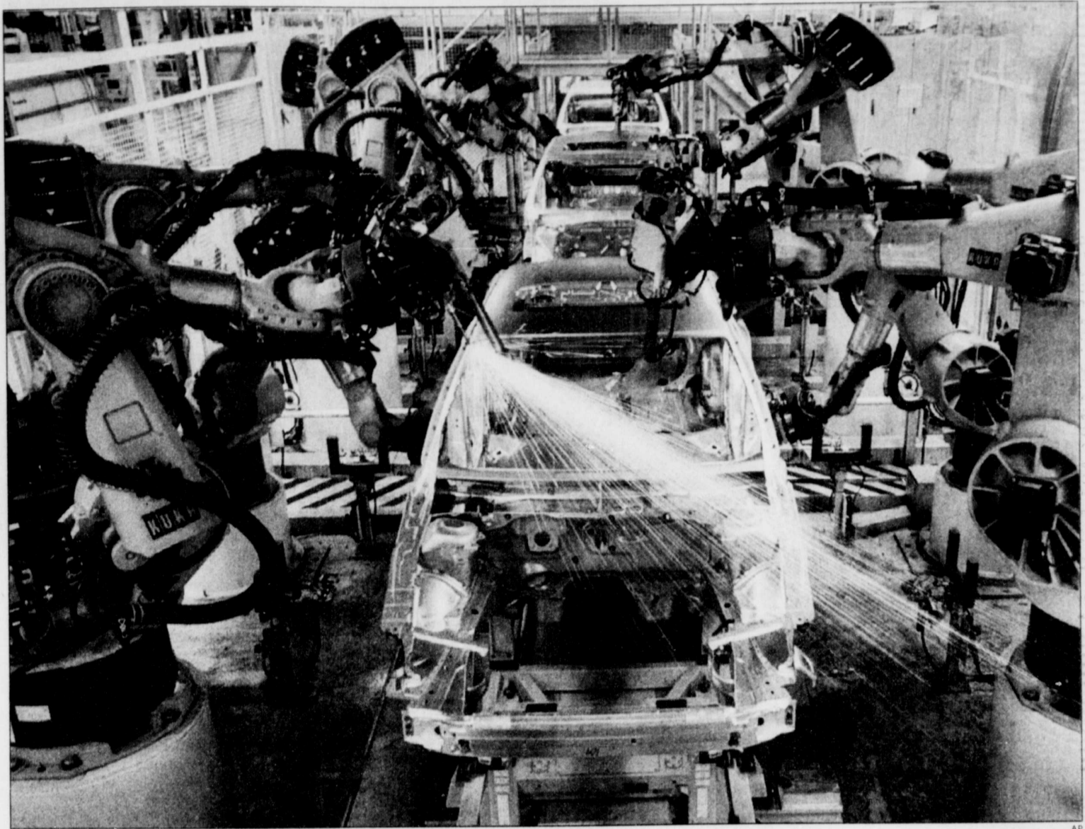
La division automobile de Volvo possède une chaîne de montage ultramoderne dans la banlieue de Göteborg, où les robots occupent une place prépondérante.
