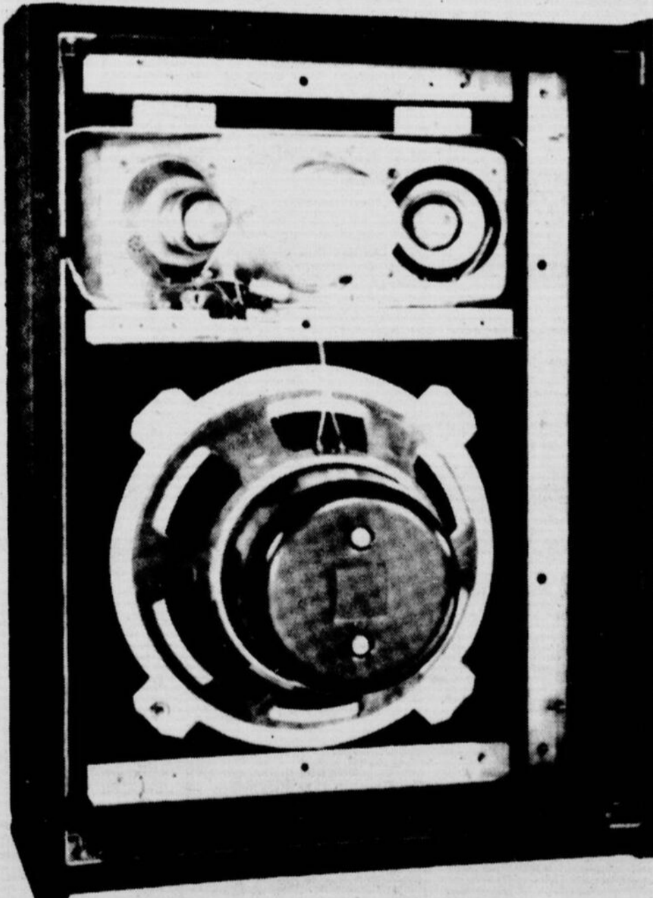
Construire un appareil aussi compliqué qu'un haut-parleur peut sembler impossible à moins d'être un expert. Pourtant, avec un minimum d'habileté et... des indications précises, vous pouvez en construire un facilement. Ou, pour être plus précis, en assembler un.
