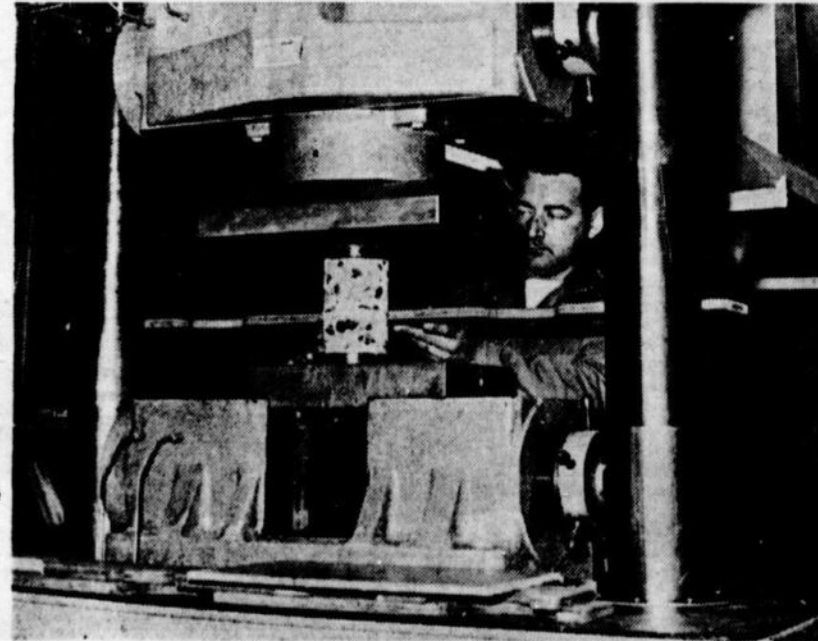
Le technicien éprouve ici, dans cette machine qui peut exercer une tension de 400,000 livres, une "carotte de béton", tirée d'un pavage ou d'un trottoir.
