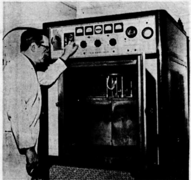
Cet appareil reproduit en 15 jours, les conditions climatiques auxquelles serait soumis un revêtement de peinture pendant une période de deux ans.
