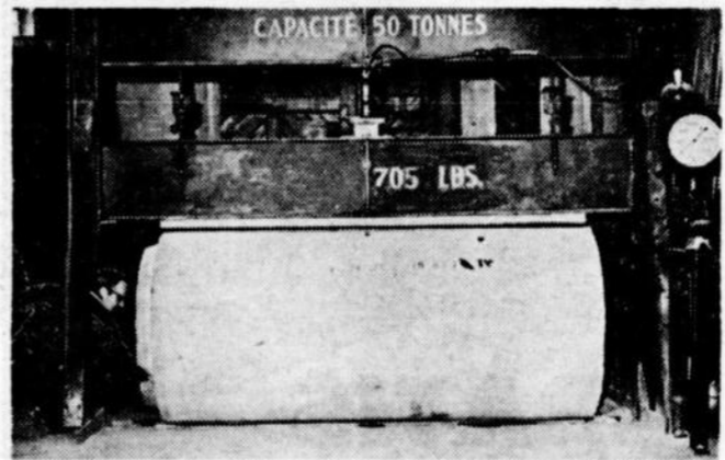
Avant de les enfouir sous terre, on s'assure toujours que les tuyaux d'égouts ne s'effriteront pas comme le "pot de terre" de la fable.
