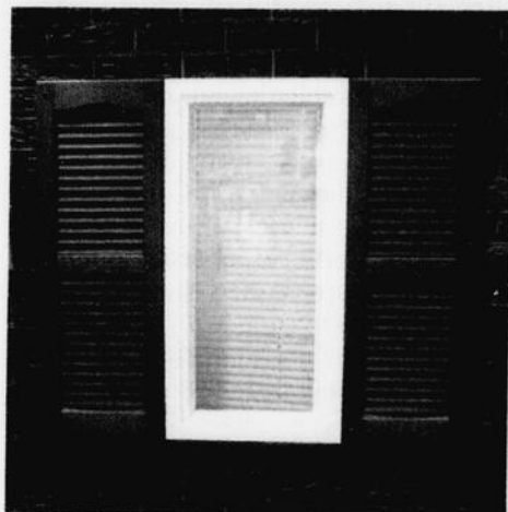
Tout en polymère : des volets sur un revêtement aux allures de brique.
