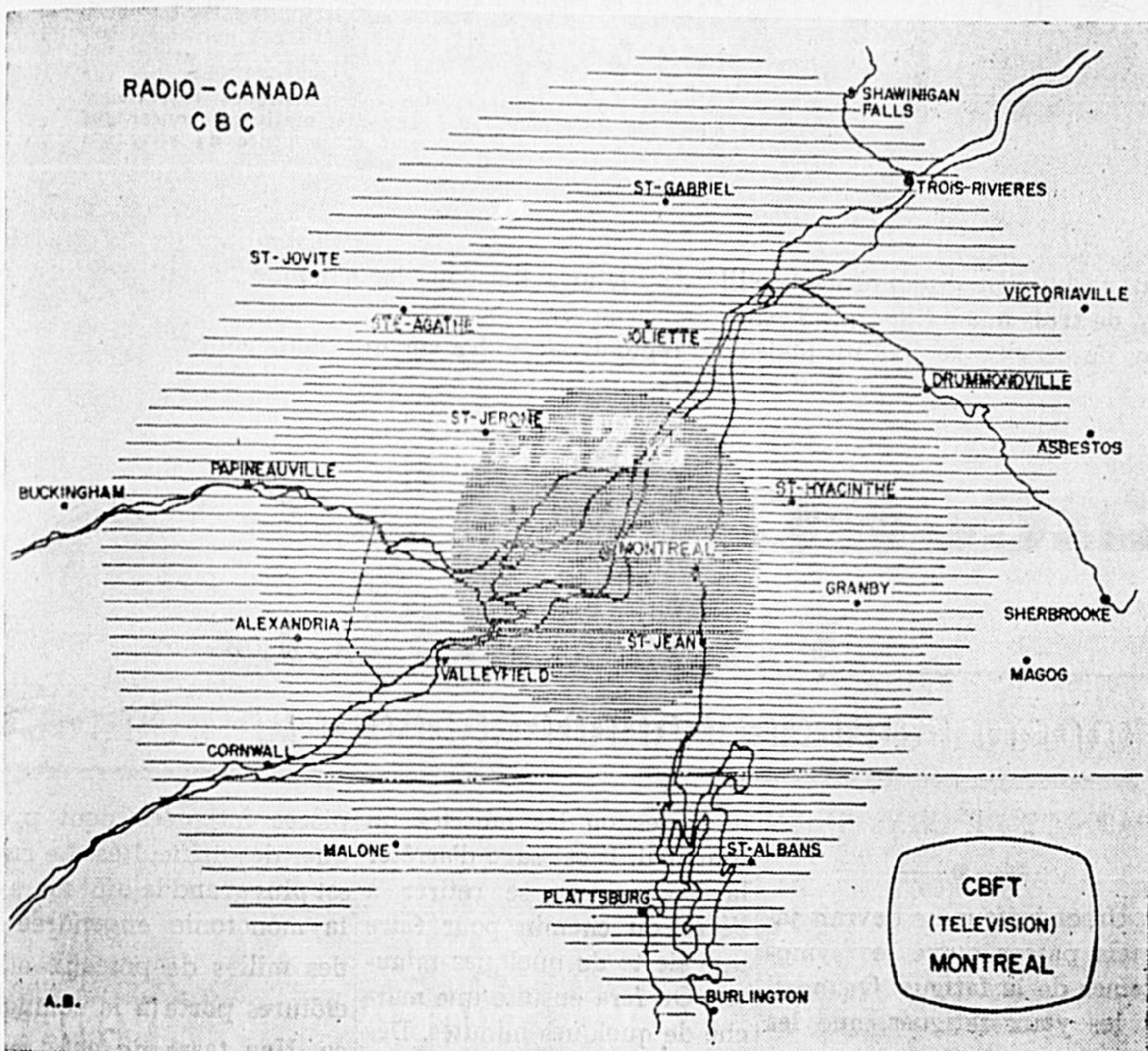
CETE CARTE représente le rayonnement approximatif du nouveau poste de télévision de Radio-Canada à Montréal, CBFT (canal 2). En réalité, les lignes de démarcations ne sont pas aussi rigides. Les ingénieurs de Radio-Canada ont tracé cette carte pour donner au public une idée approximative des trois régions où la réception sera excellente, bonne ou passable. Moins la région est ombrée, ou, en d'autres termes, plus on est loin de l'émetteur, plus grand est le besoin d'une antenne appropriée pour assurer une réception satisfaisante. Plusieurs ont déjà informé Radio-Canada que CBFT était capté parfois bien au delà de ces trois régions ombrées.
