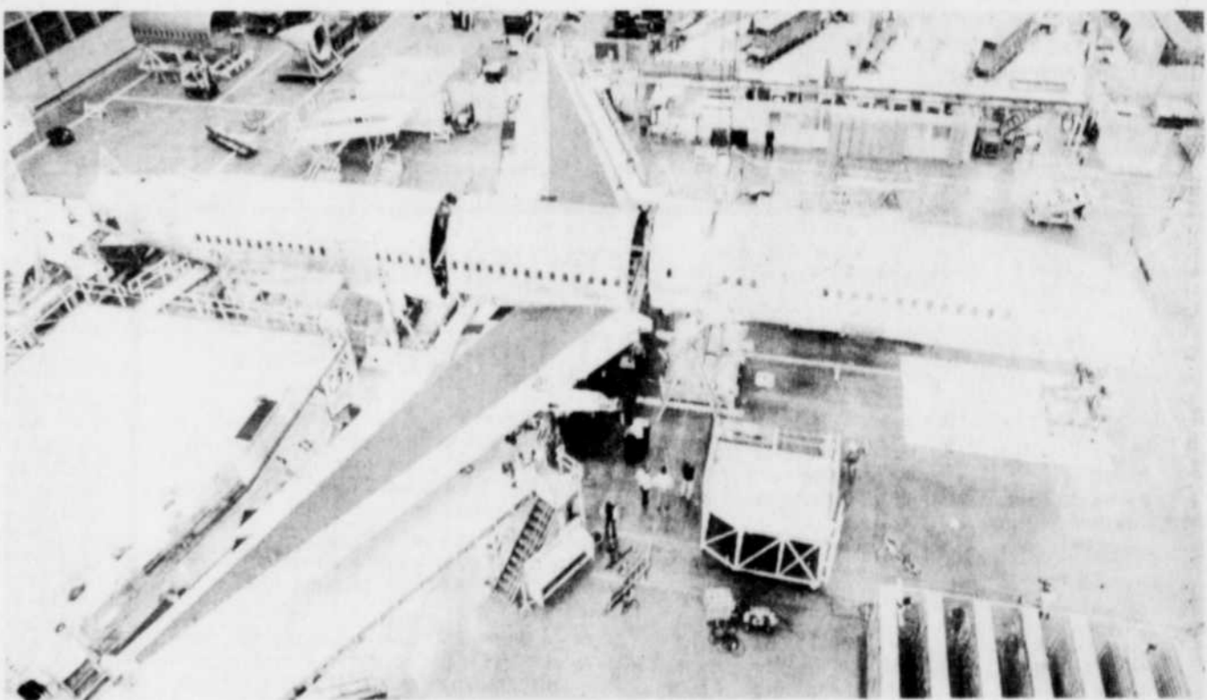
Le Boeing 757 assemblé
