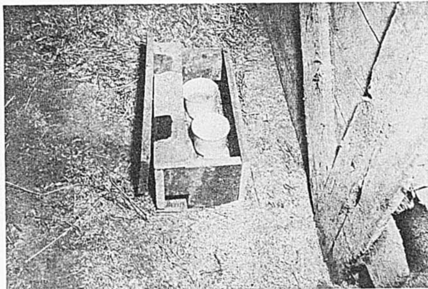
Voici l'une des installations utilisées par les autorités du Collège de Guelph au cours de leurs expériences sur les fermes de l'Ontario. L'une des boîtes contient le poison; l'autre, de l'eau. A remarquer, à gauche, le couvercle qui peut être abaissé pour éliminer tout danger pour les autres animaux.
