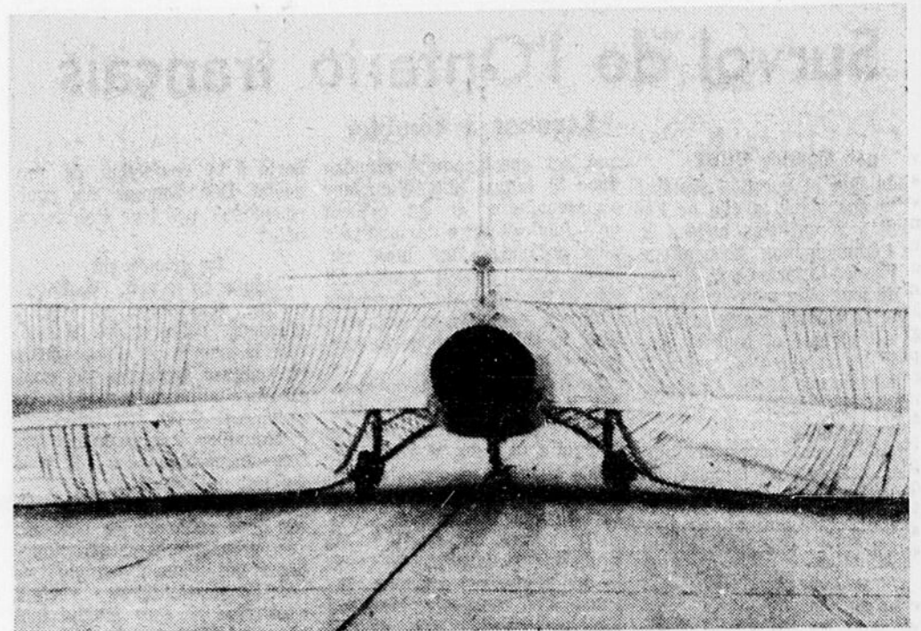
Voici une révolution dans la sécurité aérienne. Un filet de sauvetage peut recueillir les avions de ligne en cas de décollage ou d'atterrissage perturbé.
