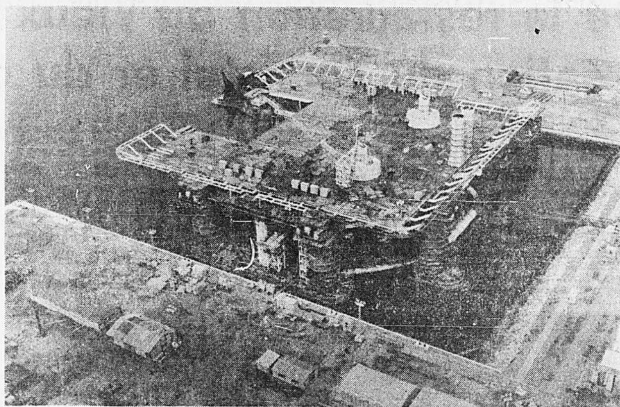
Aquapolis, la villa "maritime" de l'avenir. Les travaux de construction vont bon train, et le gouvernement japonais estime que cette ville sera le centre d'intérêt de l'Exposition d'Okinawa.
