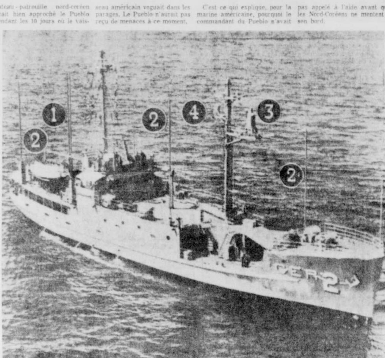
LE QUÉBÉCOIS DU NAVIRE AMÉRICAIN CAPTURÉ — Ce diagramme localise l'équipement extérieur du patrouilleur de la U.S. Navy, "Pueblo" devant servir à recueillir l'information pour l'"Intelligence" américaine. Le Pueblo a été capturé par les forces Nord-Coréennes lundi soir. (1) Antennes jumelles qui indiquent la direction des signaux captés afin que d'autres appareils puissent se
