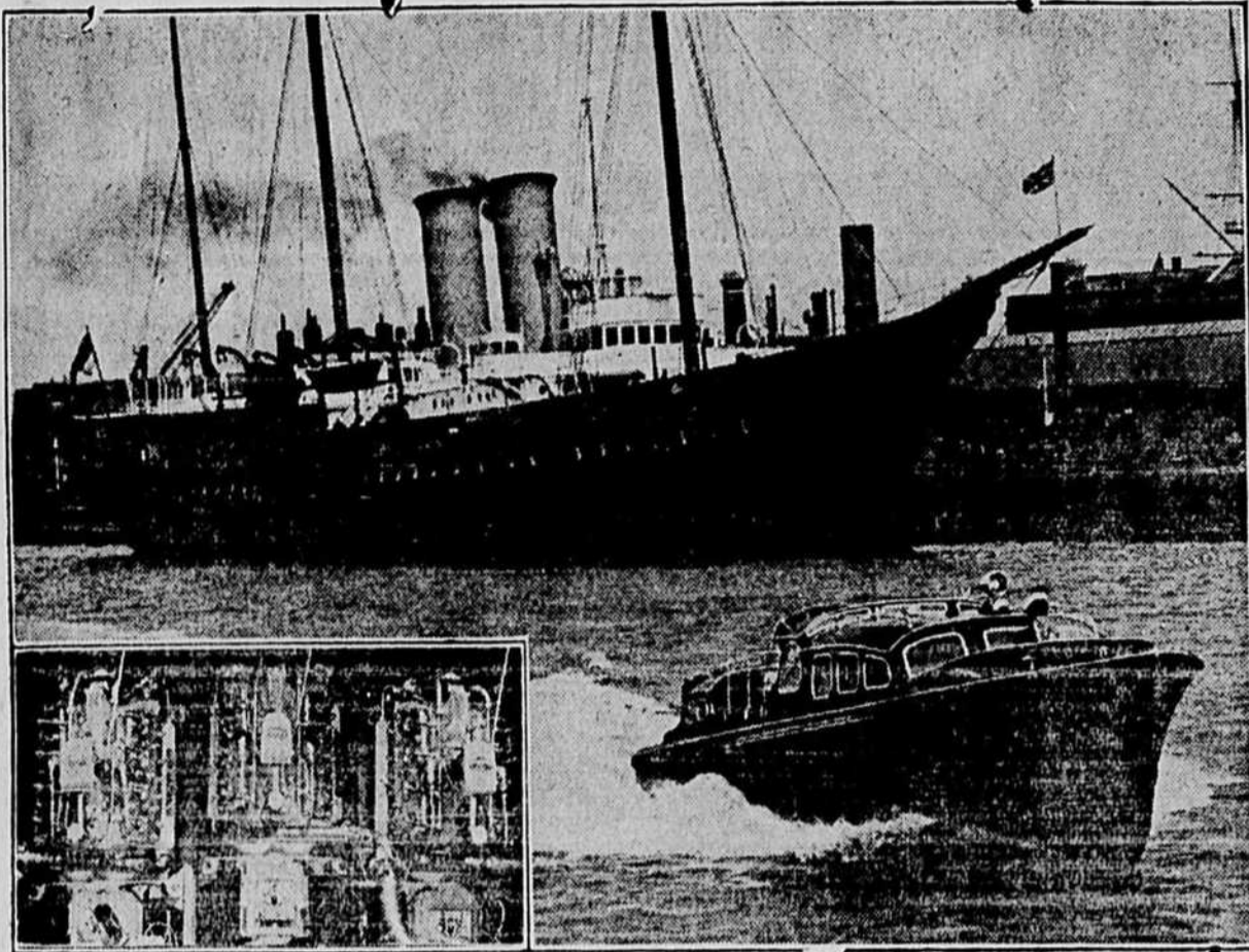
Voici le croiseur fabriqué pour Leurs Majestés le Roi Georges VI et la Reine Elizabeth. Nous le voyons ici avec, au second plan, le yacht royal. Ce croiseur pourra filer 20 nœuds à l'heure, et à 16, son moteur sera silencieux. Il est mû par 3 moteurs du type Ford V-8. Long de 40 pieds, il pourra répondre à toutes les exigences royales.
