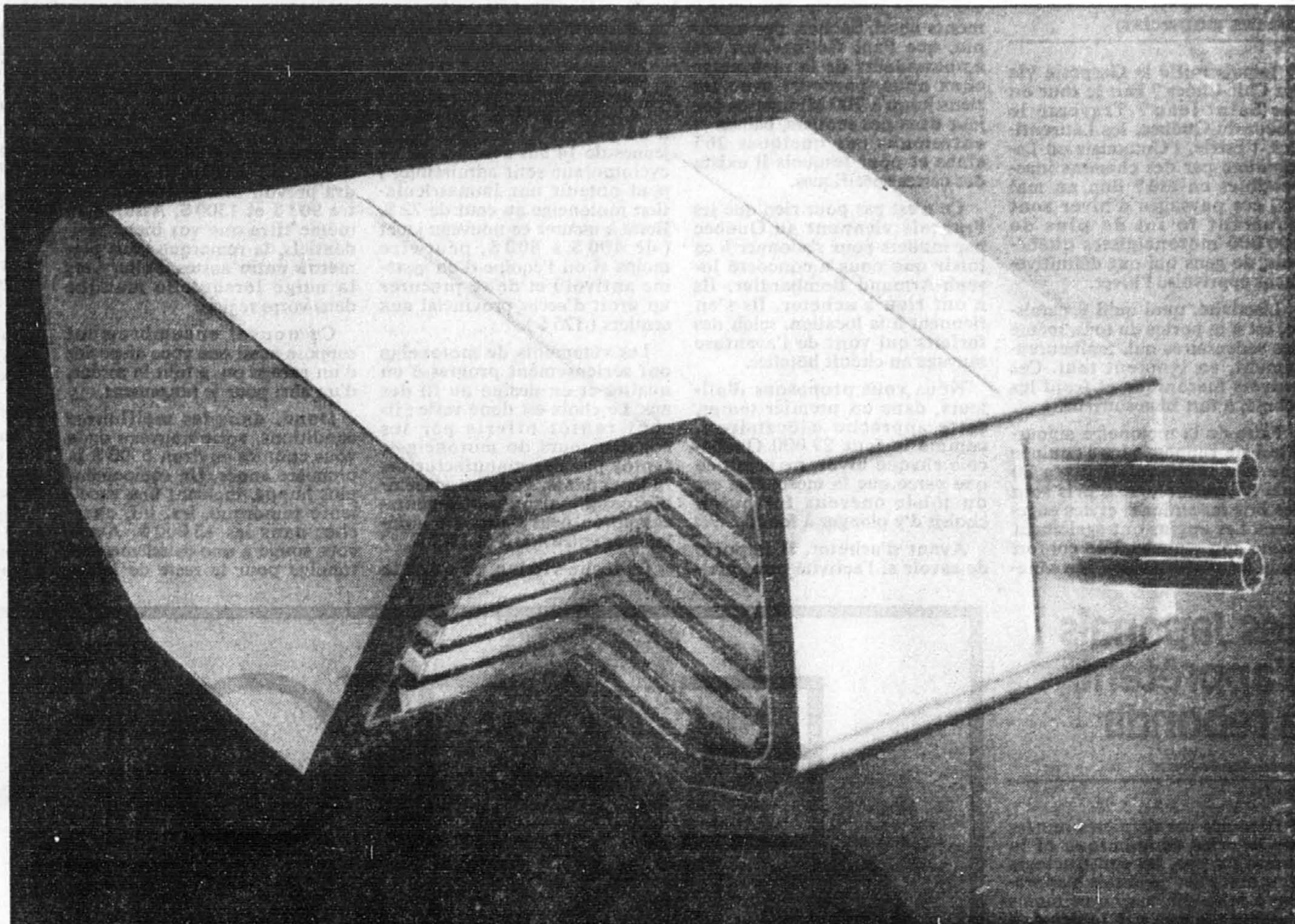
Dans ses voitures de la nouvelle Série 5, BMW propose un radiateur de chaleur latente qui entrepose de la chaleur pendant plusieurs jours. Ceci permet de réchauffer la cabine et de désembuer les vitres en peu de temps l'hiver.
