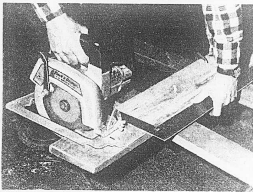
L'équerre de métal permet à la scie de faire une coupe parfaite.
