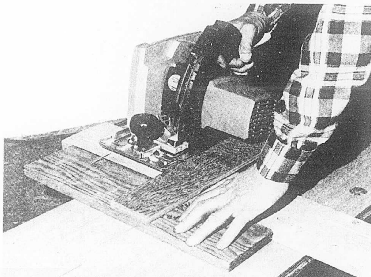
L'équerre de bois, rainurée au point de coupe, est facile à utiliser et donne un résultat excellent.
