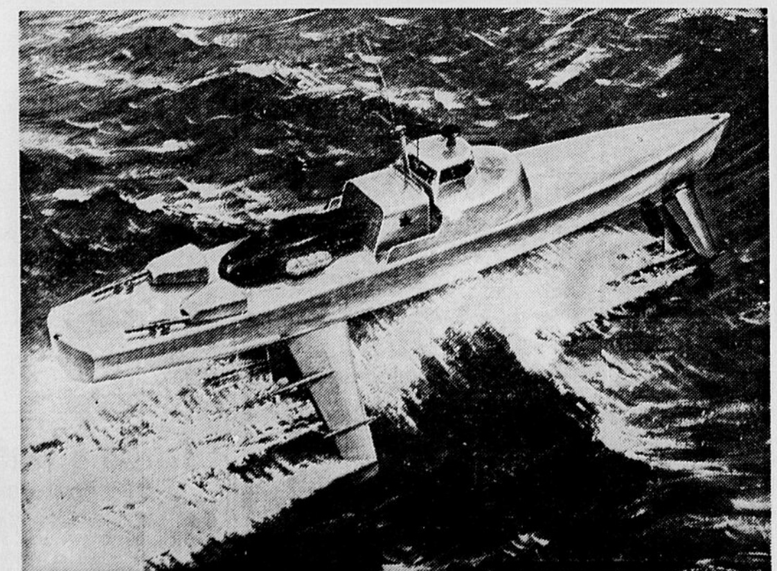
Voici un sketch du prototype de l'hydroglisseur qui va être conçu et réalisé pour la Marine royale du Canada. On prévoit que la vitesse de cette embarcation de 150 pieds sera de 50 noeuds et plus. Ce projet est la conclusion de recherches intensives entreprises par le Canada à Toronto, en est le principal entrepreneur; d'autres industries canadiennes contribuent également à la réalisation de ce projet. (Photo Défense Nationale)
