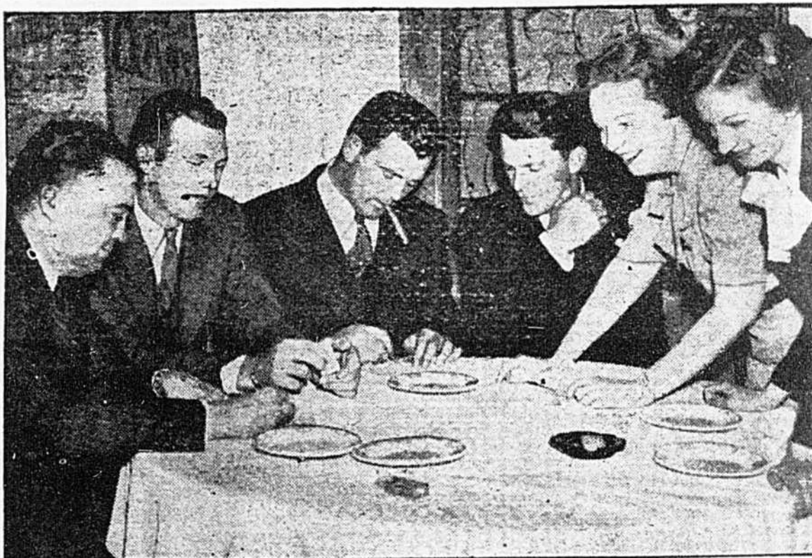
Les champions du monde n'ont pas tardé à célébrer leur victoire, et on voit un groupe de ceux-ci oubliant leurs soucis de la série mondiale dans un club de nuit du Manhattan. De gauche à droite: J. Edgar Hoover, chef des "G-Men"; Bill Dickey, Jimmy Braddock, champion du monde à la boxe et George Selkirk. Les deux jeunes filles qui apparaissent ici sont en quête d'autographes.
