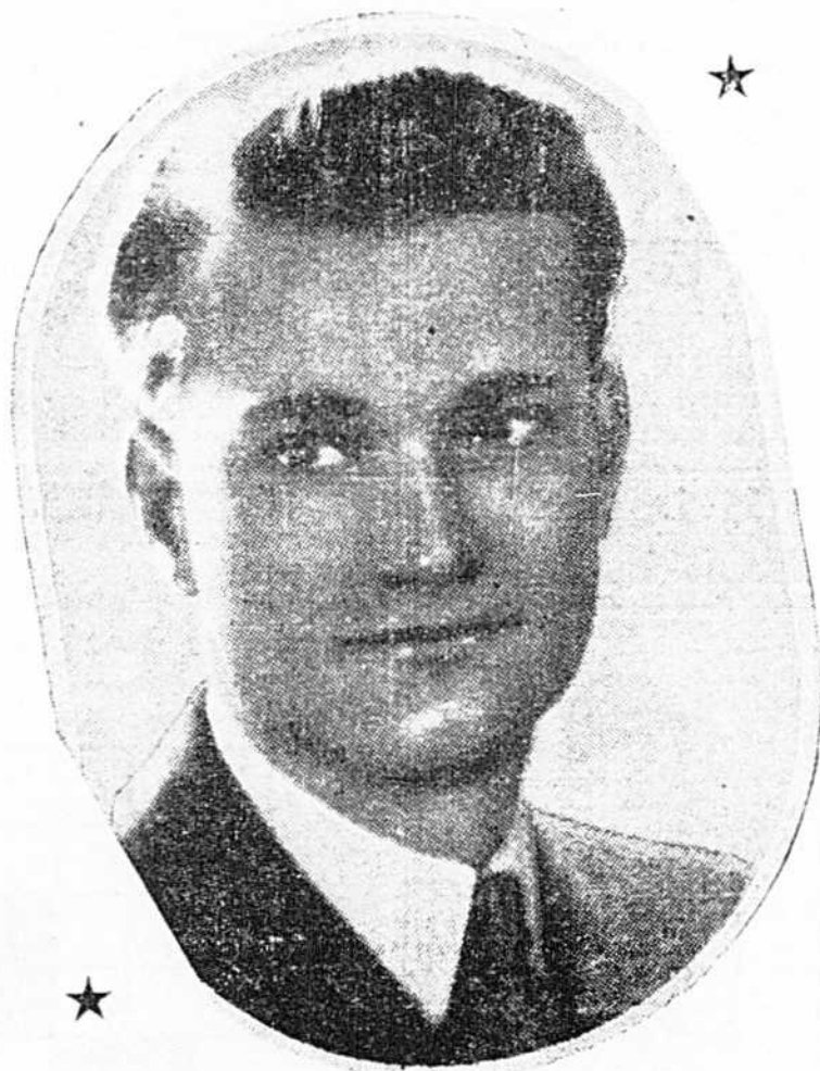
Le populaire "RED" SKELTON qui a été engagé une quatrième fois pour remplir les fonctions de maître de cérémonies sur la scène du Loew's. On pourra le voir cette semaine à ce dernier théâtre aux côtés du chanteur Morton Downey et plusieurs autres
