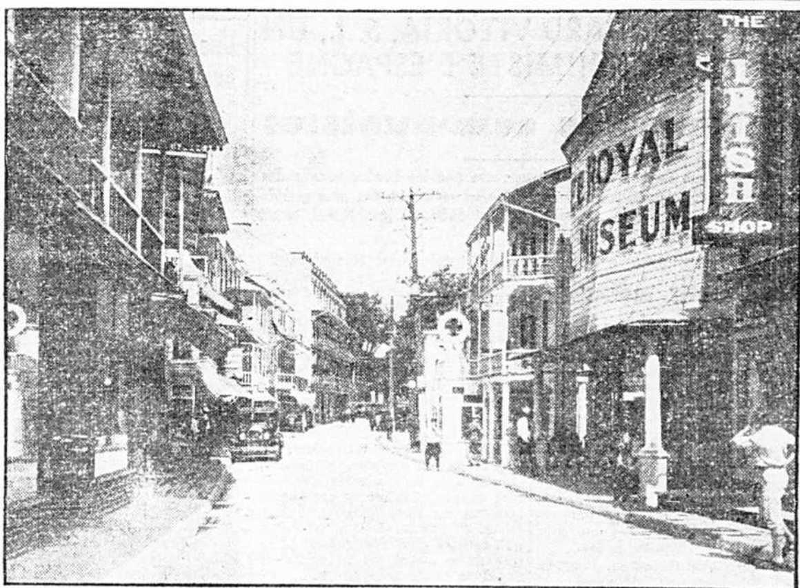
Voici un aspect du quartier de Ste-Anne de Beaupré qui a été ravagé par les flammes, hier. A gauche, au premier plan, l'hôtel Columbus, et à l'arrière, les hôtels du Musée, Windsor, et au bout de la rue, l'hôtel Morel; à droite, l'Irish Shop, le Musée Royal, les deux restaurants d'un M. Lacroix. Le sanatorium est situé au bout de cette avenue, à droite. (Photo Chemins de fer national du Canada.)
