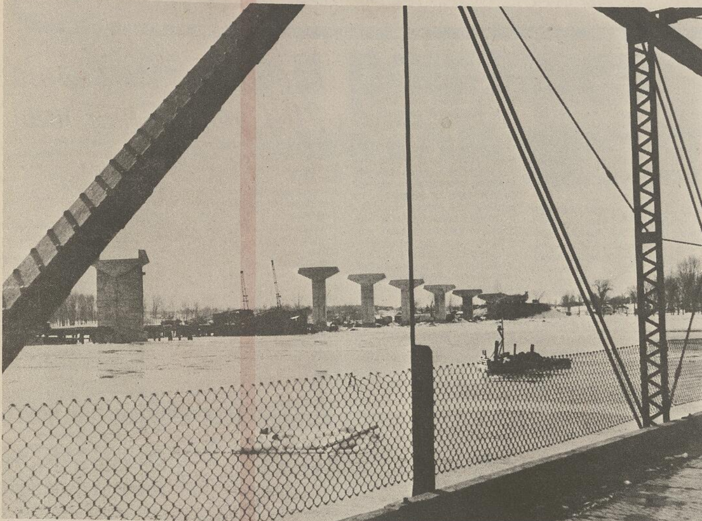
LES TRAVAUX du nouveau pont qui enjambe la rivière Richelieu entre Candic et Noyan progressent normalement. Ce nouveau pont sera vraisemblablement ouvert à la circulation au cours de l'hiver 1969-70. C'est la firme J.A. Levasseur, de Montréal, qui a obtenu le contrat de l'ordre de $2,500,000.
