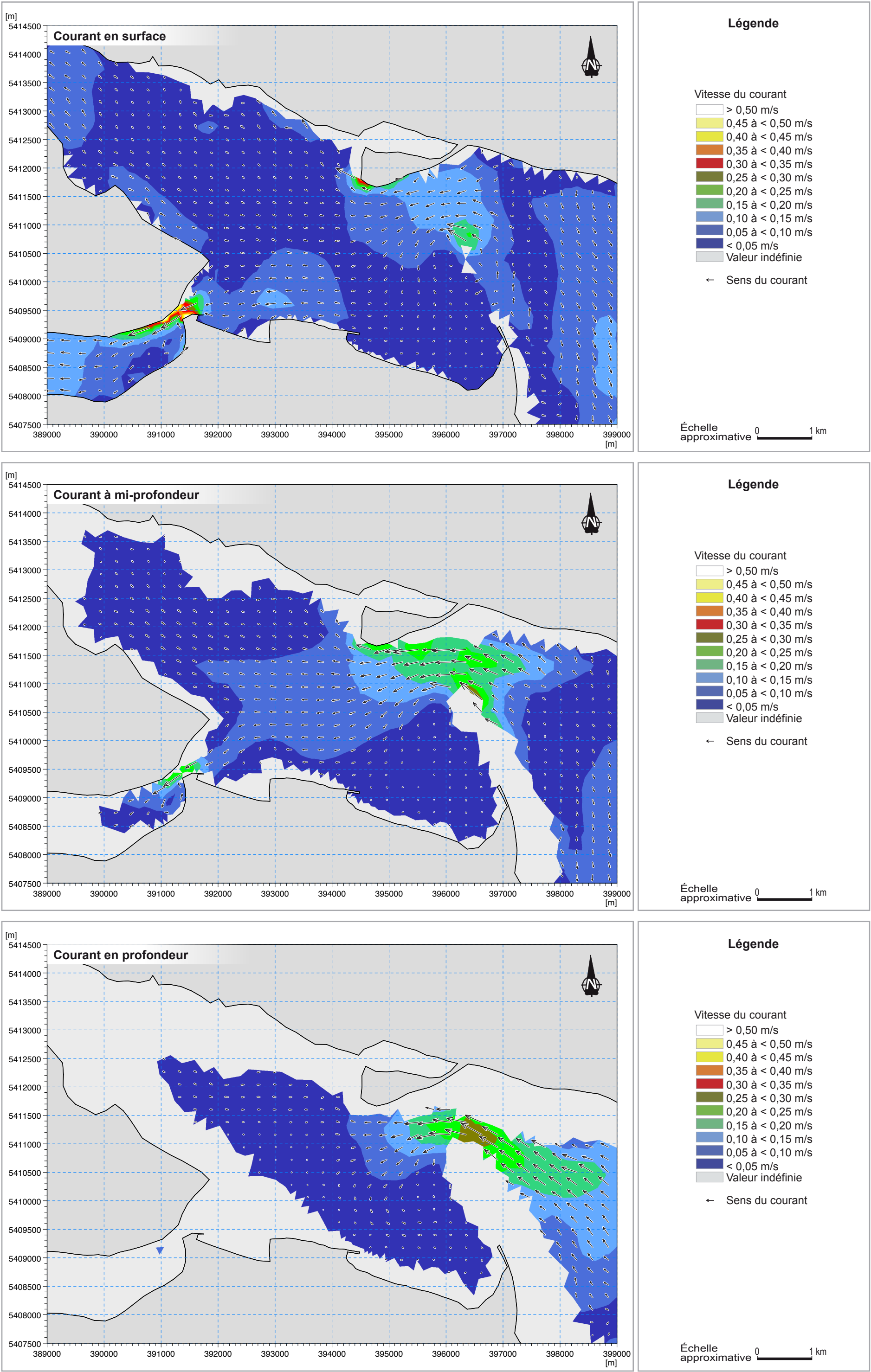
Figure 4A Simulation de base – Courants maximums à marée montante
