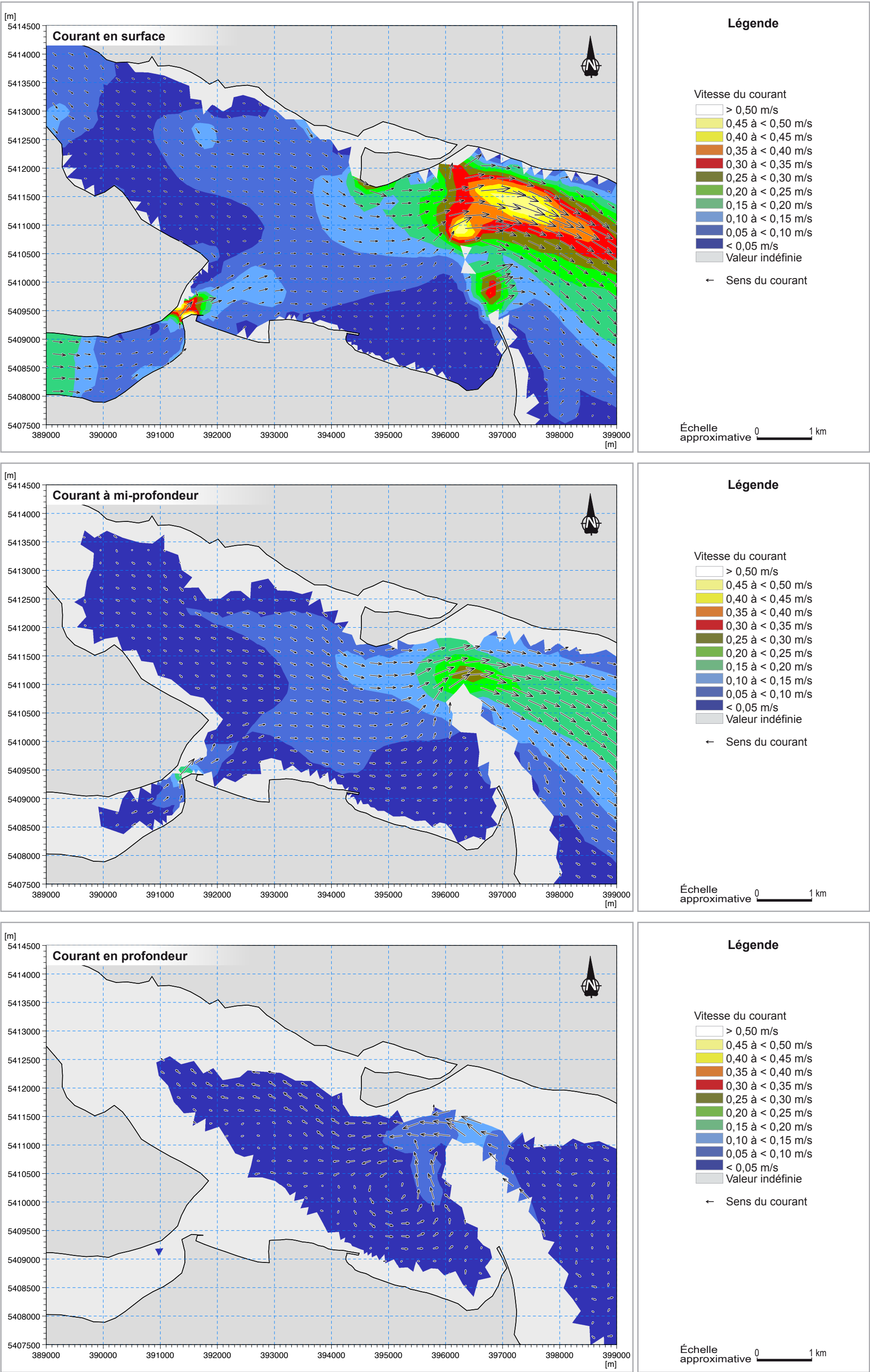
Figure 4B Simulation de base – Courants maximums à marée descendante
