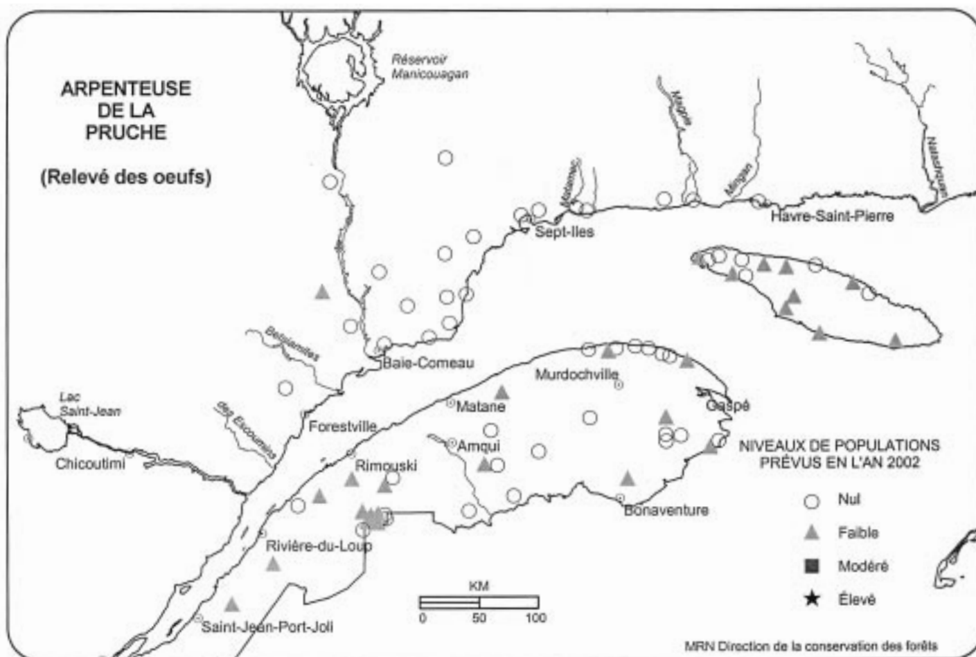
Carte 5 – Niveaux de populations d'arpenteuses de la pruche prévus en 2002
