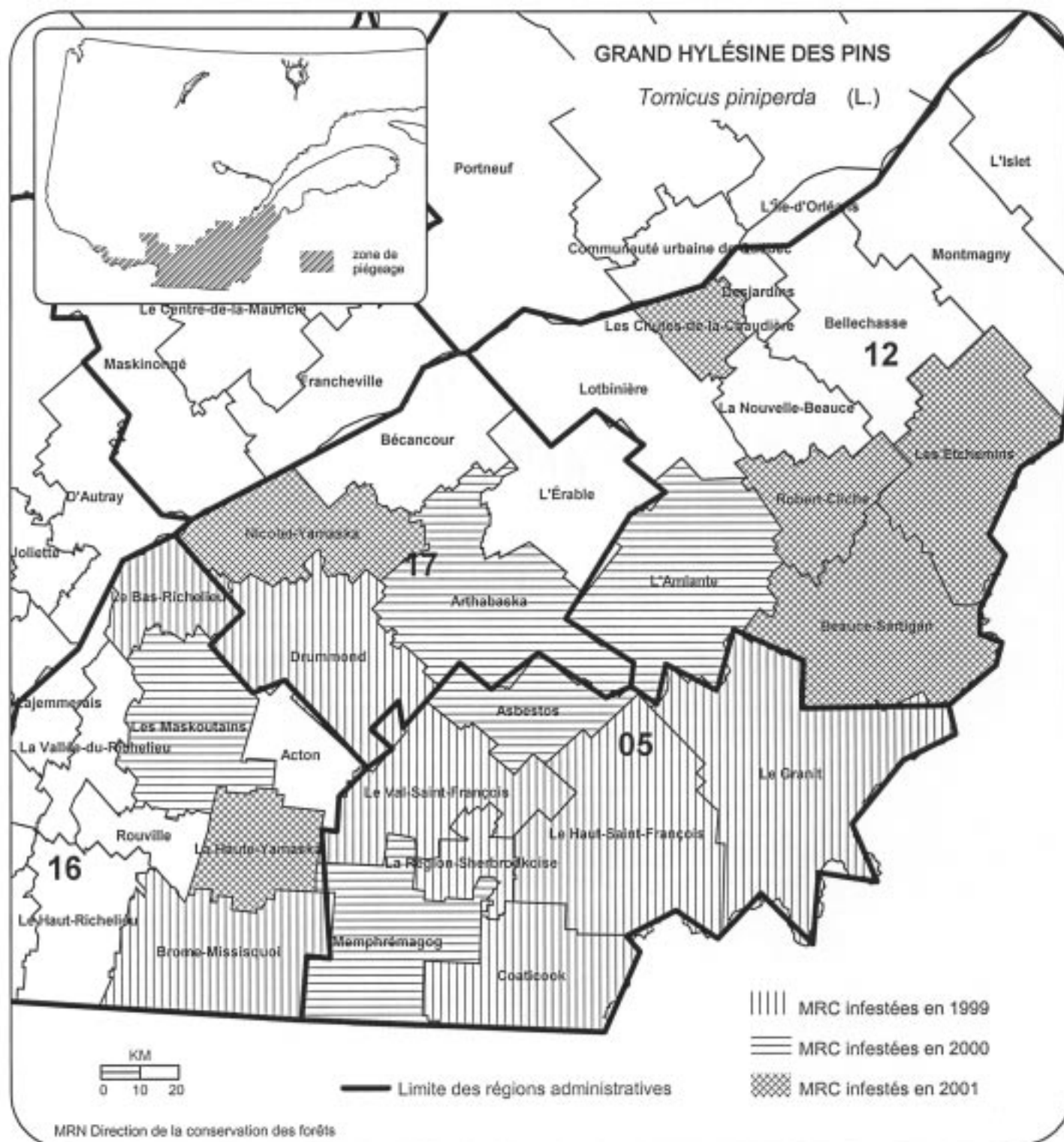
Carte 8 – Distribution du grand hylésine des pins au Québec, en 2001
