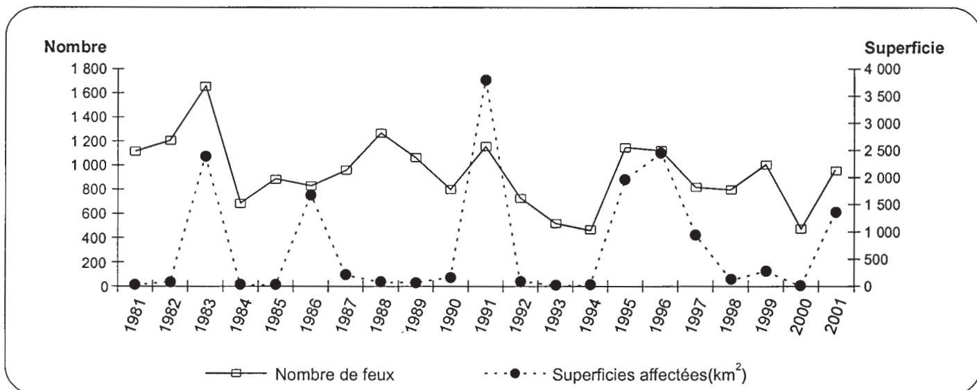
Figure 2 – Nombre de feux de forêt répertoriés et superficies affectées, de 1981 à 2001
