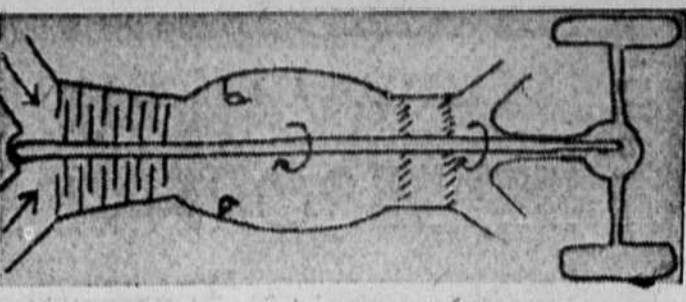
Principe toujours très simple. L'air entre à l'avant. Le compresseur le précipite dans la chambre de combustion. De là il agit sur la turbine à ailettes et sort par les deux manchettes. En passant par la turbine, il la fait tourner à 28.000 tours par minute et l'axe ainsi entraîné agit à la fois sur le compresseur et sur l'engrenage (dans la boîte arrière) et, par entraînement, sur les deux roues. Dans le turbopropulseur, l'action est identique sauf que l'axe entraîne une hélice à l'avant au lieu des roues à l'arrière et que les gaz sont utilisés comme puissance de réaction.
