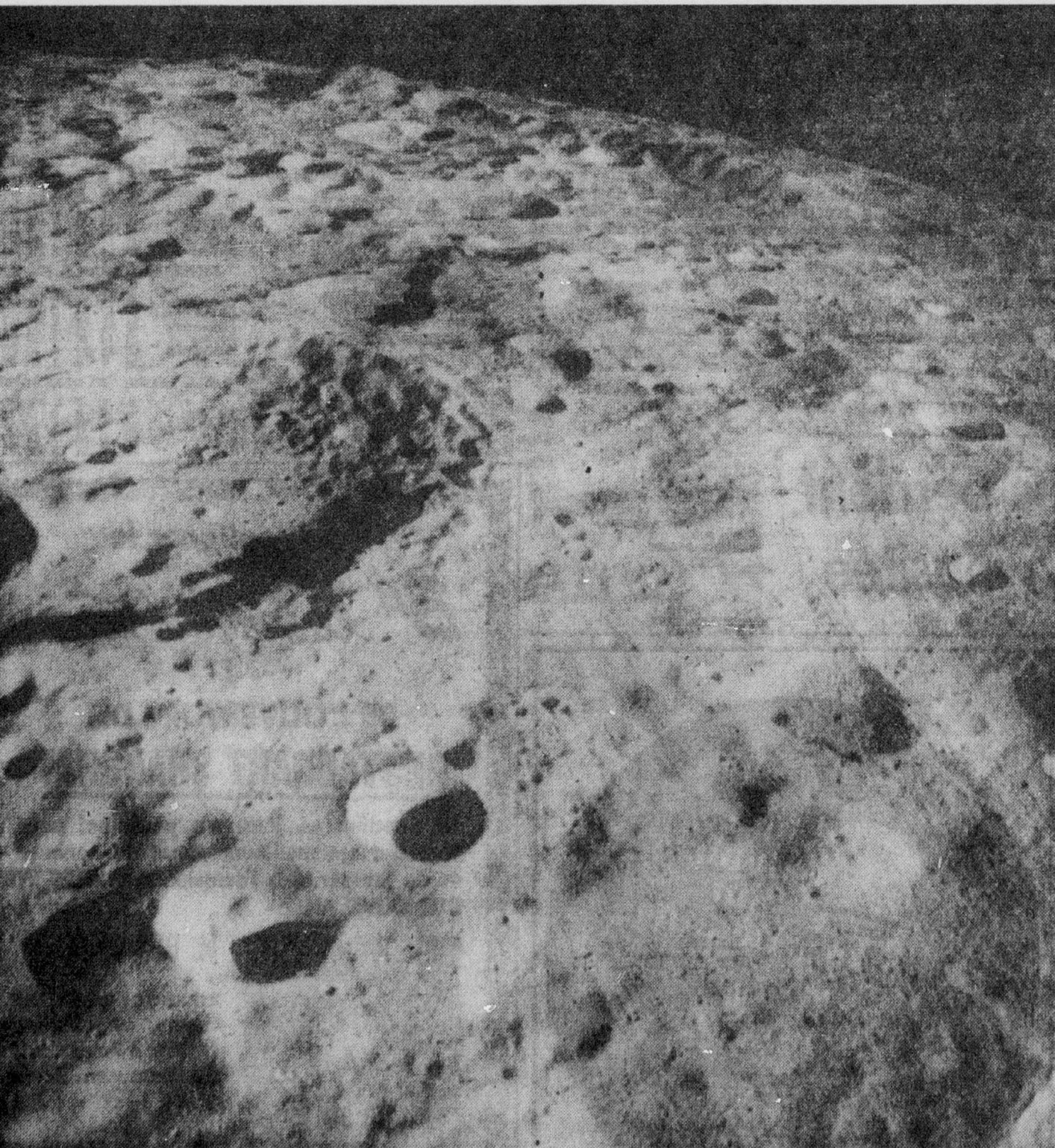
LA LUNE VUE DU VEHICULE SPATIAL — Cette photo a été prise de la cabine spatiale Apollo-8 à l'aide d'un téléobjectif orienté au sud en direction du large cratère Coclennius. On y remarque quelque chose de neuf : le ruisseau qui en traverse le bord. Le groupe de trois cratères est composé, lui, des cratères Magelhaens, Magelhaens A et Colombo A. Le cratère Coclennius est situé à la latitude : 10 degrés sud, à la longitude : 45 degrés est, et a environ 40 milles de diamètre.
