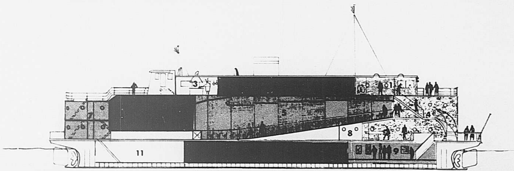
1. Entrée, guichets, vestiaire 2. Restaurant 3. Cuisines 4. Foyer et bar 5. Salle du théâtre 6. Scène 7. Loges, cabines 8. Toilettes 9. Salon projeté 10. Machines 11. Loges des comédiens.
