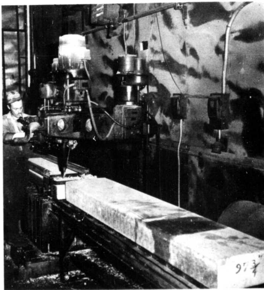
AVANT L'ASSEMBLAGE, M. Roméo Painchaud perce des trous dans les barres avec une perceuse électrique. Ces trous serviront à attacher les électrodes à la barre omnibus.
